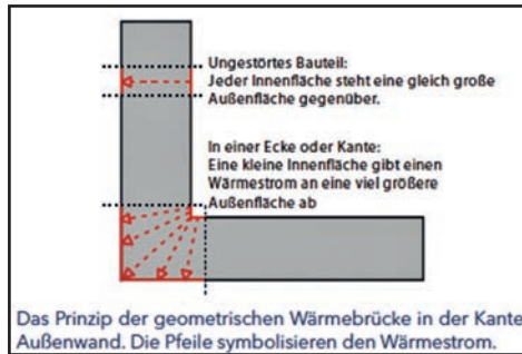
Das Prinzip der geometrischen Wärmebrücke in der Kante Außenwand. Die Pfeile symbolisieren den Wärmestrom.
