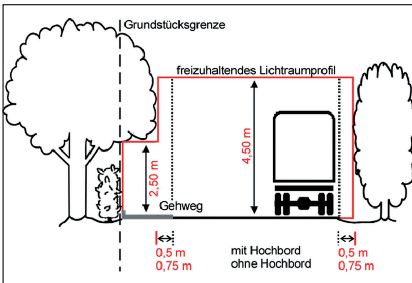
Lichtraumprofil
