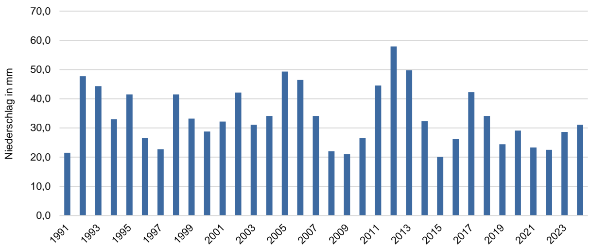
Höchstwerte des Tagesniederschlages im Zeitverlauf von 1991 bis 2024
