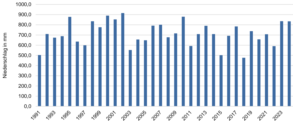
Jahresniederschlagsmenge im Zeitverlauf von 1991 bis 2024
