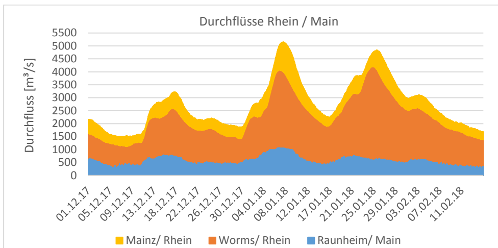
Abb. 29: Durchflüsse in Rhein und Main
