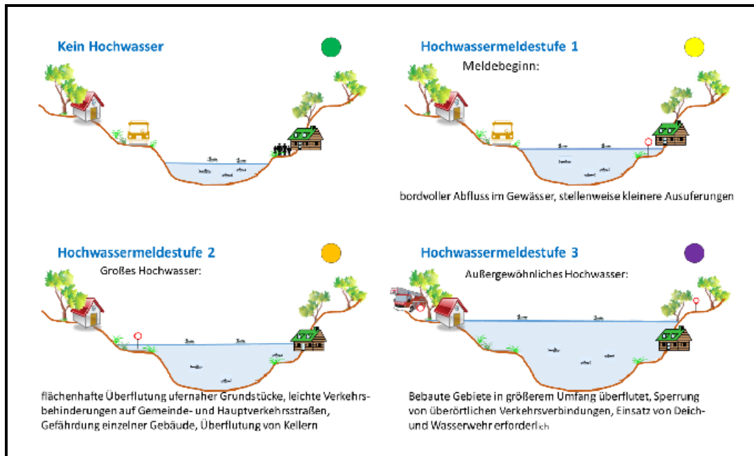
Abb. 7: Hessische Hochwassermeldestufen
