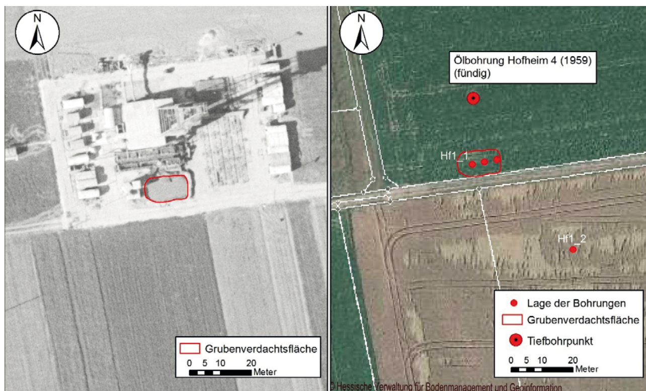
Abb. 4: Bohrplatz der Erdölbohrung Hofheim 4 (links) (HVBG 2018d, Flug Nr. 769/59; Bild Nr. 7210; Flugdatum 13.04.1959, verändert) und aktuelles Luftbild mit ungefährender Lage der Bohrpunkte und einer Verdachtsfläche (rechts) (HVBG 2018a; HLNUG 2018b)
