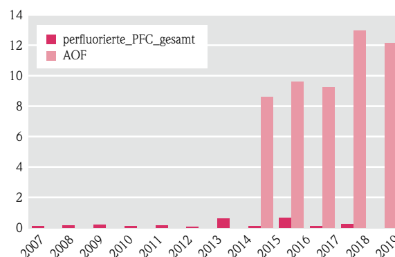
Abb. 1: PFC-Messungen im Schwarzbach bei Astheim – die dunklen Säulen zeigen den Parameter „perfluorierte_PFC_gesamt“, die hellen Säulen den Summenparameter „AOF“
