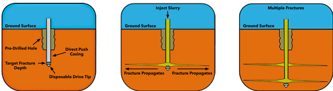
Abb. 1: Darstellung des Funktionsprinzips von ISCO mit Fracturing
