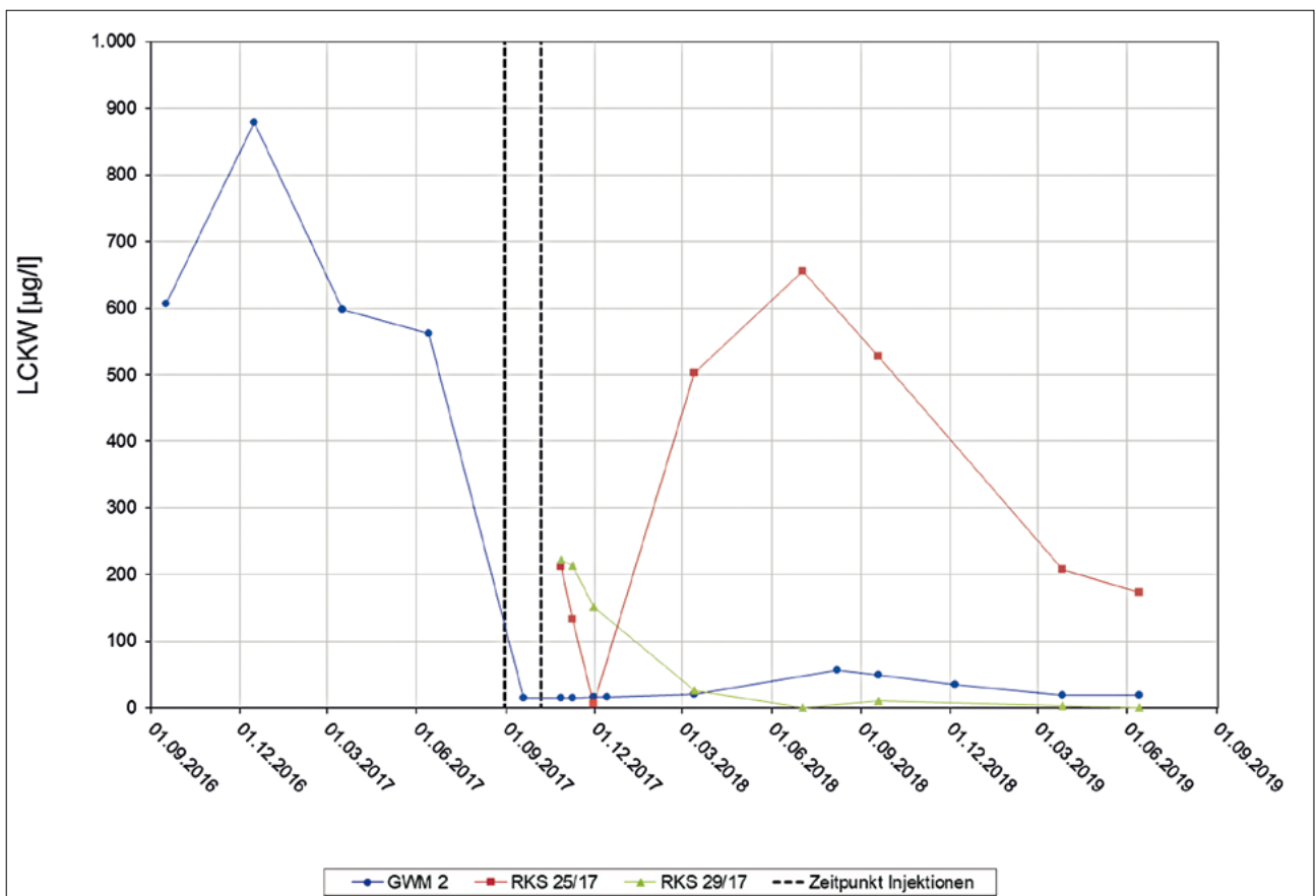
Abb. 3: Verlauf der LCKW Konzentrationen im Bereich des Pilotversuches; die gestrichelten vertikalen Linien zeigen die Zeitpunkte der Injektionen
