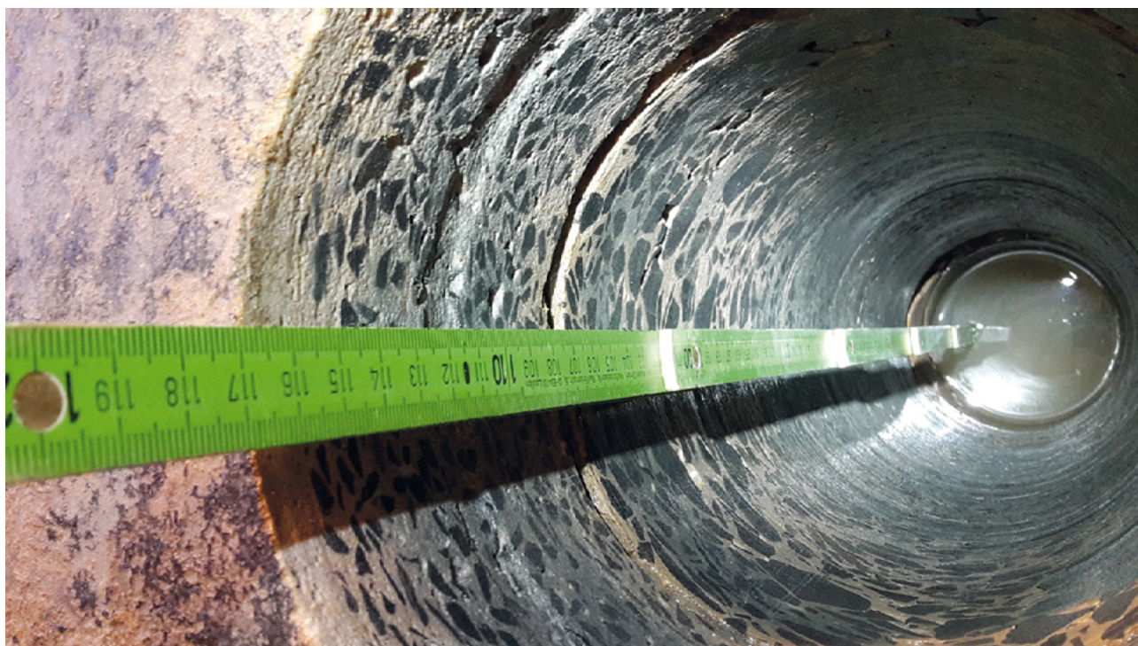
Abb. 2: Durchörterte Bodenplatte in einem Altgebäude
