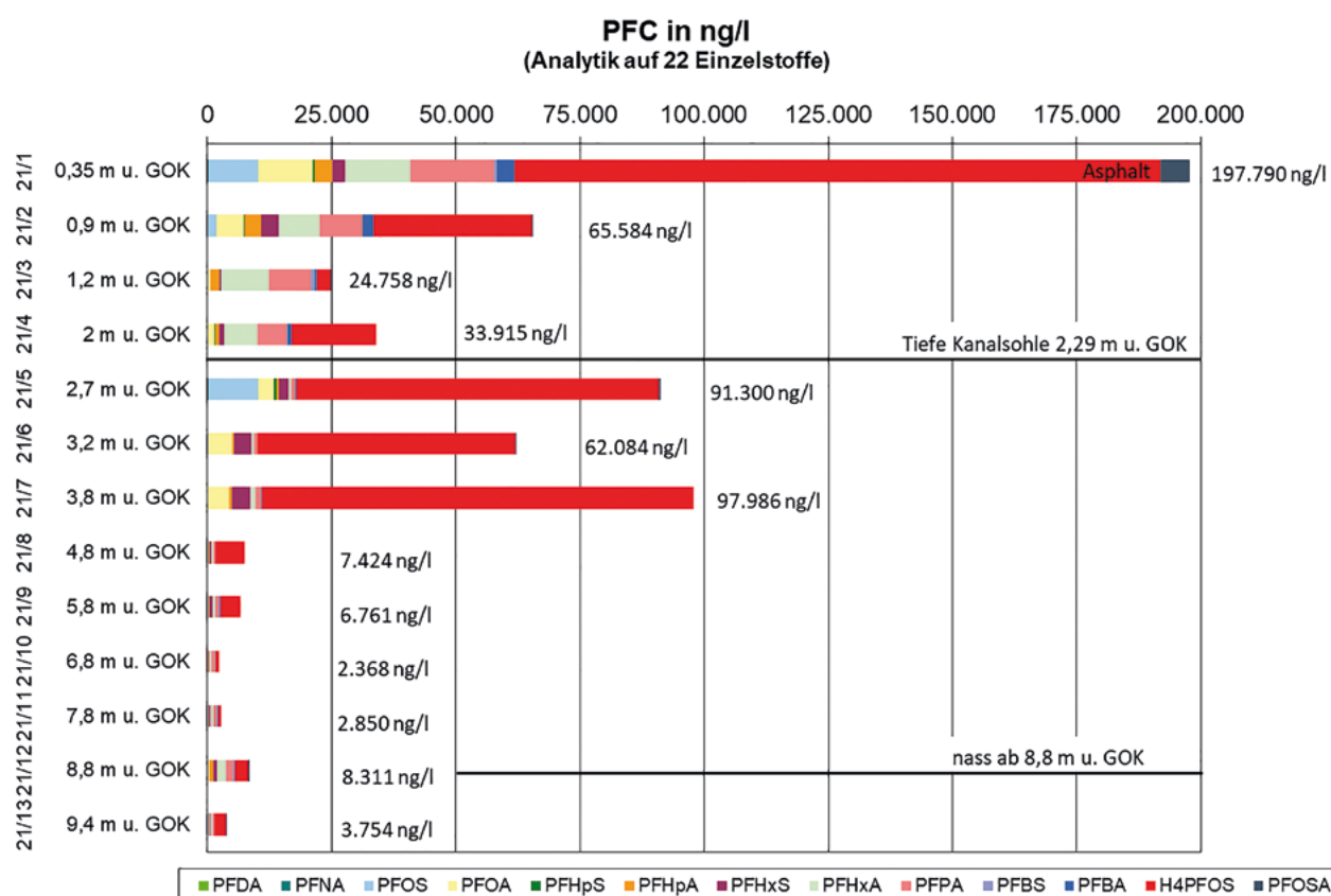
Abb. 3: Ergebnisse der tiefenorientierten PFC-Untersuchung im 2:1-Eluat aus einer Sondierung auf dem Standort einer Feuerwache
