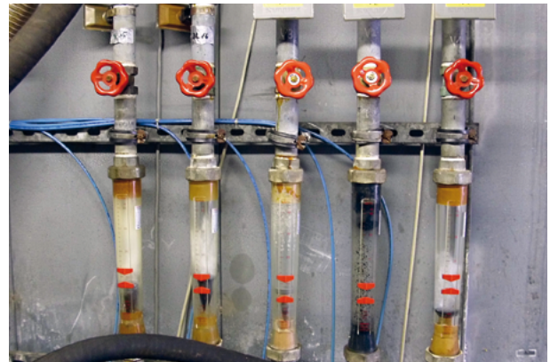
Abb. 8: Fallbeispiel 4 – Schwebedurchflussmesser mit Wasser und ausgeschwemmter Aktivkohle
