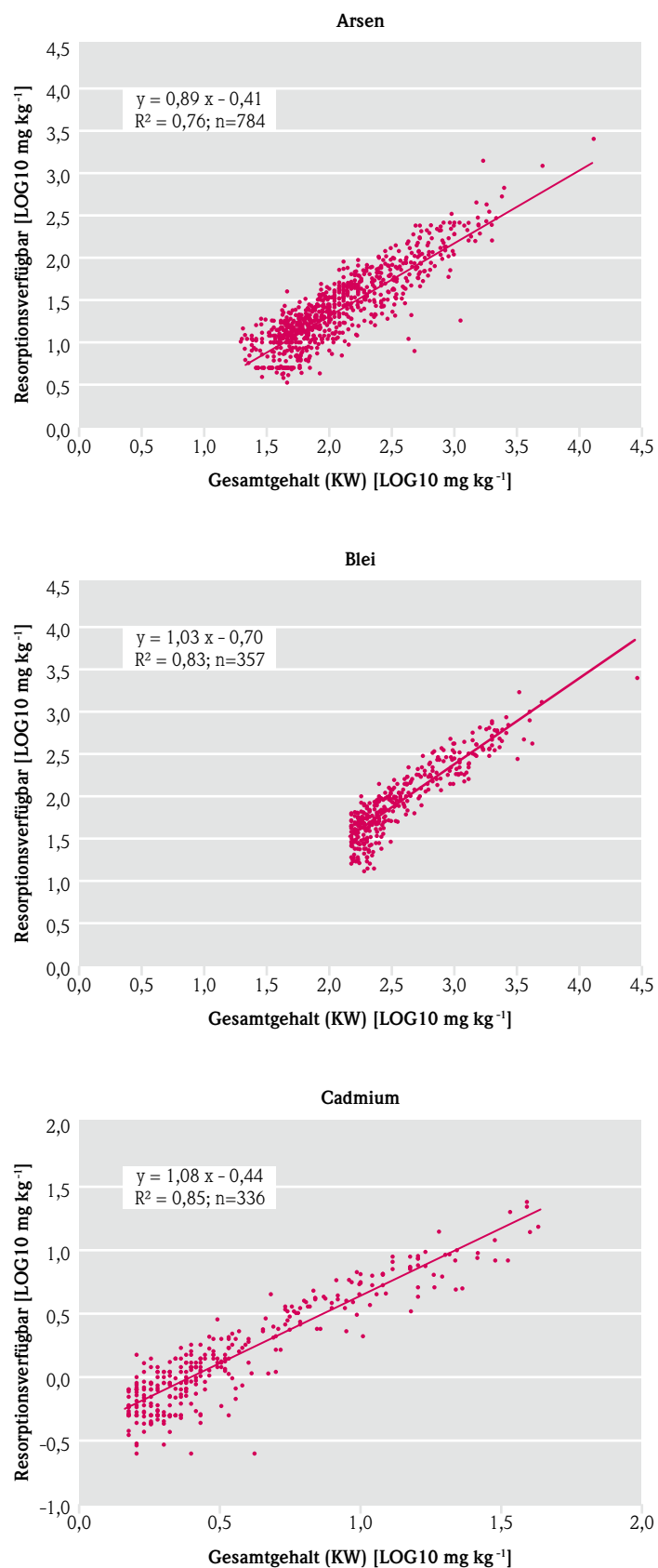
Abb. 4: Logarithmierte Werte für As, Pb und Cd
