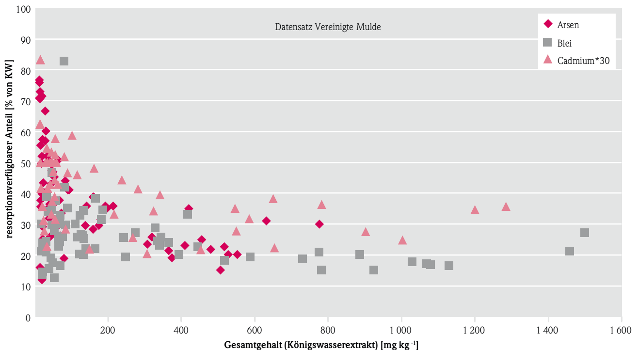
Abb. 2: Resorptionsverfügbarer Anteil für As, Pb und Cd in Abhängigkeit vom Gesamtgehalt (Datensatz Vereinigte Mulde)
