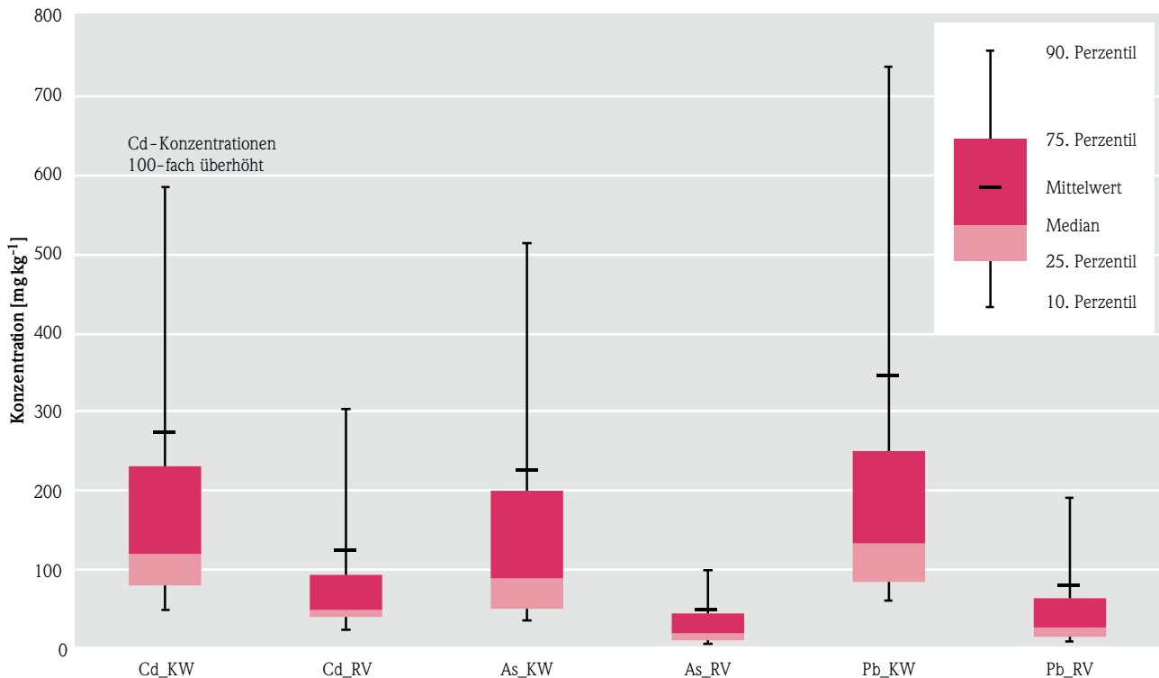
Abb. 1: Vergleich der Gesamtgehalte (KW) und der resorptionsverfügbaren Gehalte (RV) für Cd, As und Pb im Oberboden/ LfULG Sachsen, FIS Boden – Auswertung 15.05.2019
