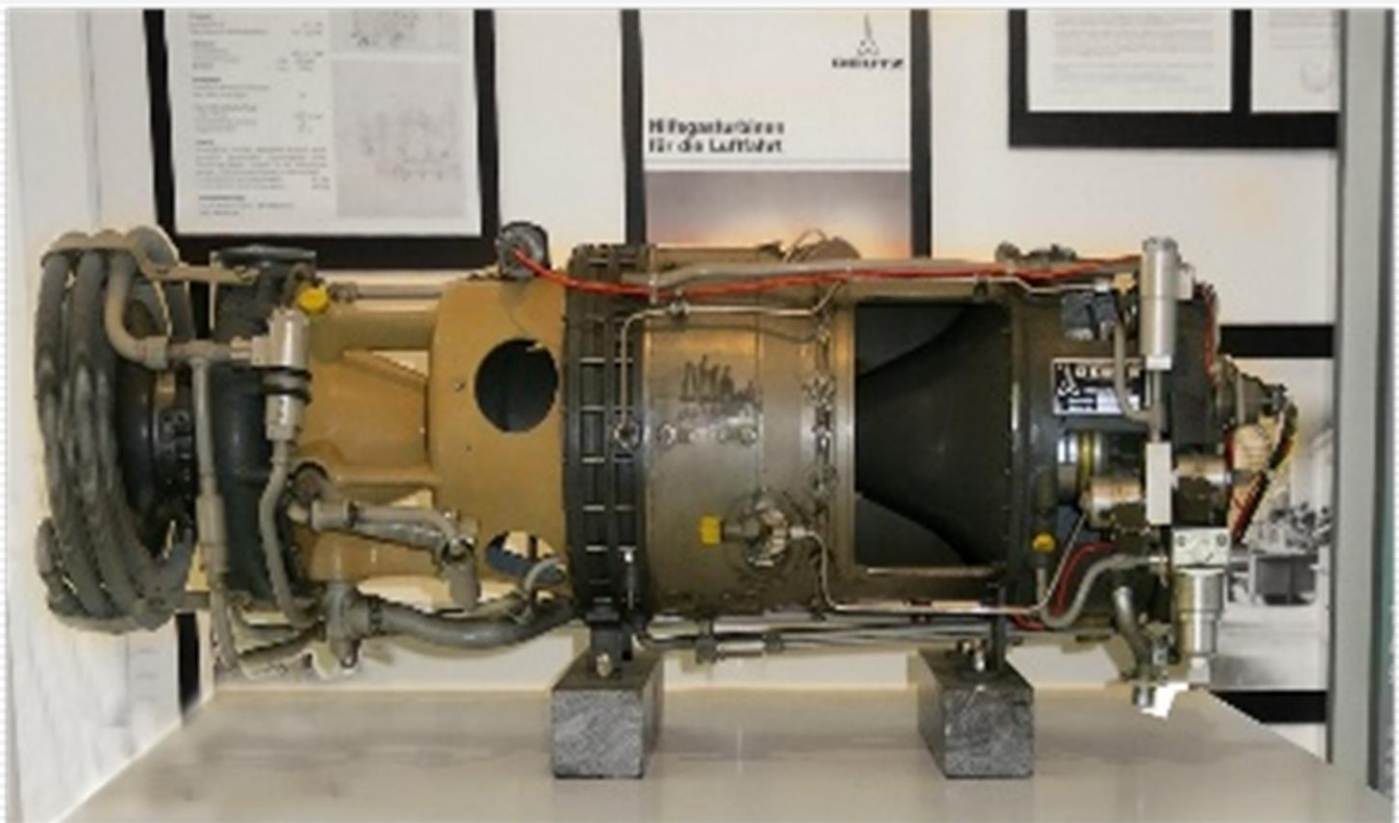
Der Einwellen-Luftlieferer KHD T212
