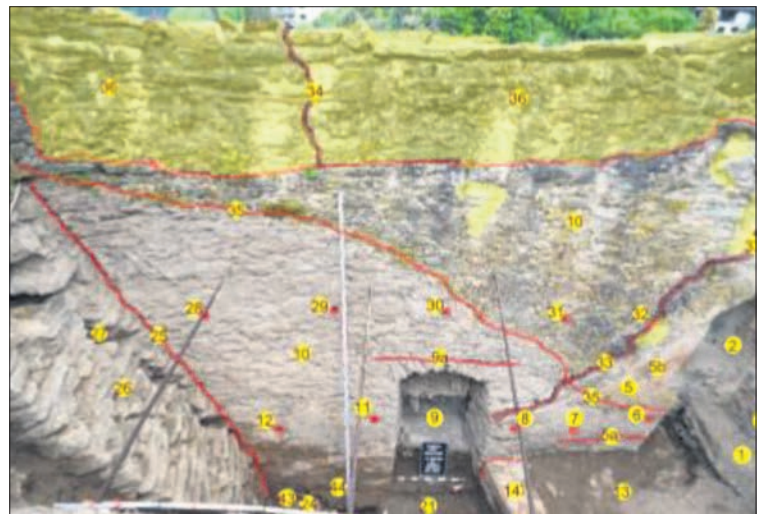
Die Linien zeigen, wie die Risse die Mauer durchziehen. Foto: Stadt Eppstein
