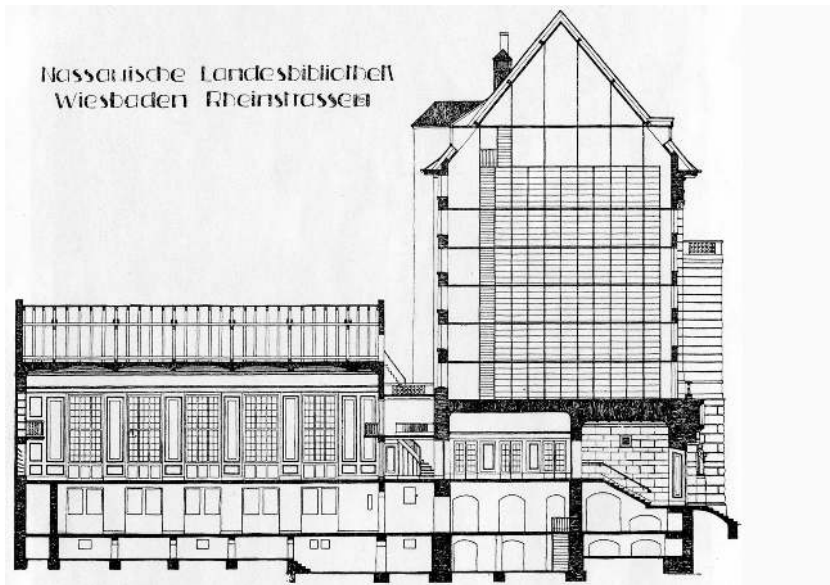
Abbildung 6.6: Längsschnitt durch den Lesesaal und das Eingangs-Treppenhaus
