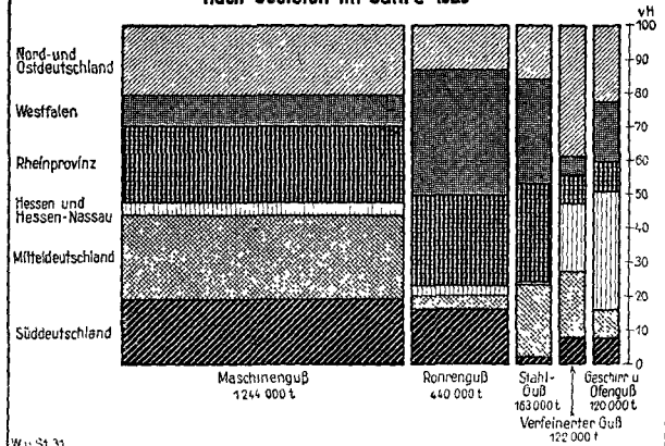
Die Herstellung der wichtigsten Gießereierzeugnisse nach Gebieten im Jahre 1929
