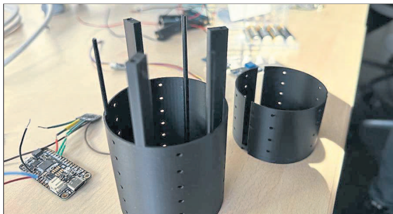
Das ist das Gehäuse des Satelliten. Es ist etwas größer als eine Getränkedose und alle Komponenten müssen in dem Behälter Platz finden.
