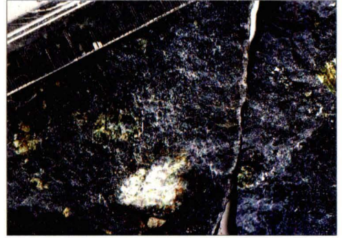
Abb. 7: Basalt vom Hörkopf (grau) mit Olivin (grünlichgelb)
