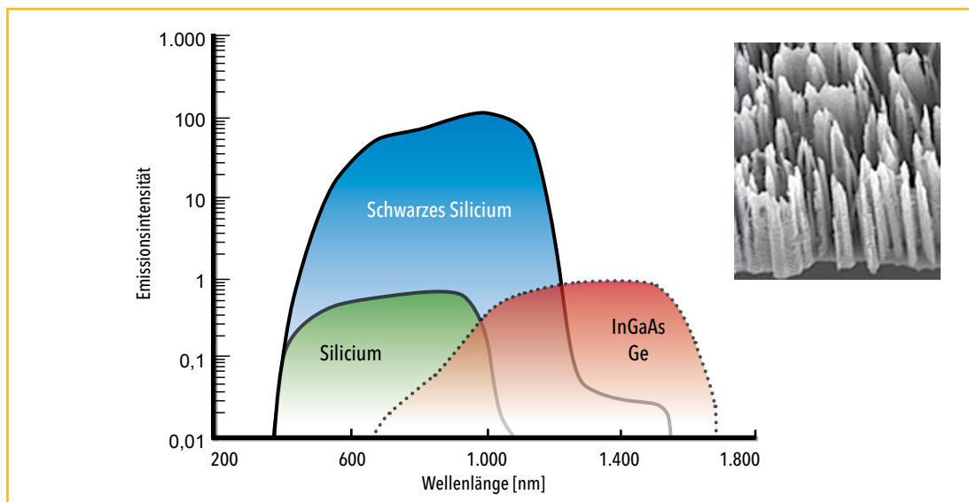
Empfindlichkeitsspektrum eines „Black Silicon“-Sensors
