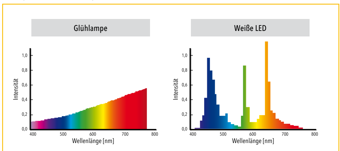
Lichtspektren einer Glühlampe und einer weißen LED
