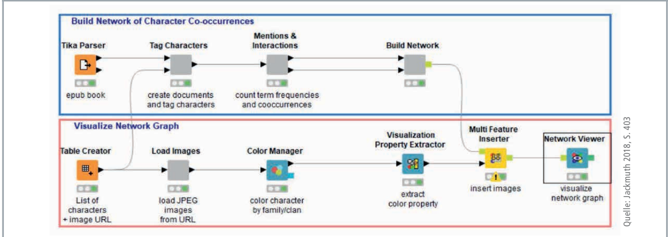
Abb. 02: Ausschnitt aus dem KNIME-Workflow
