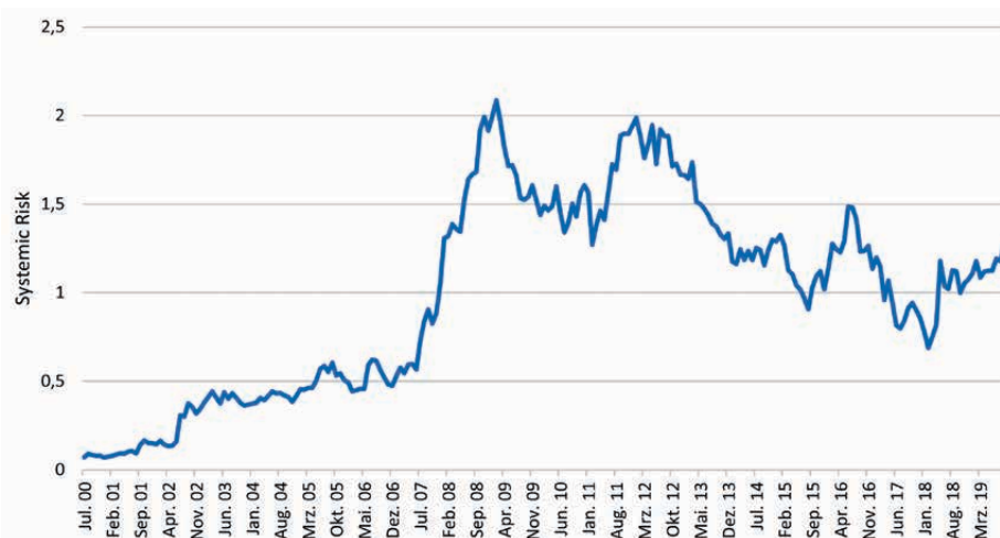
Abb. 01: SRISK-Systemrisikomessung
