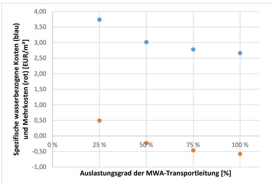
Abbildung 13: Spezifische wasserbezogene Kosten (blau) und Mehrkosten (rot) [in EUR/m 3 ] der Betriebswasserversorgung aus Mainwasser in den Günthersburghöfen in Abhängigkeit vom Auslastungsgrad der MWA-Transportleitung
