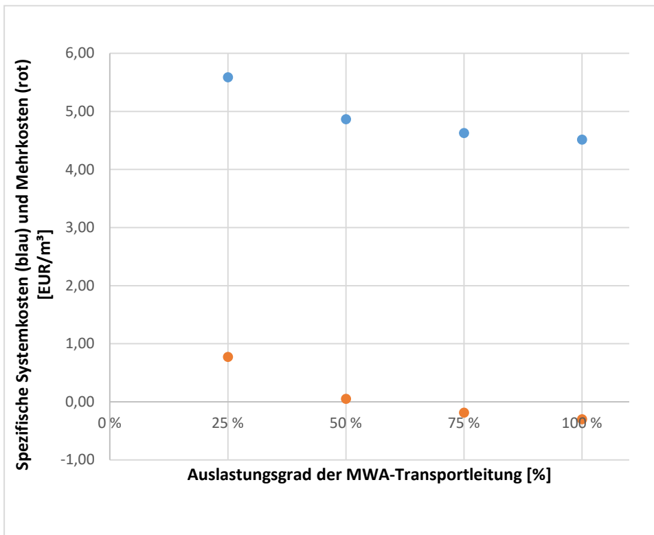
Abbildung 12: Spezifische Systemkosten (blau) und Mehrkosten (rot) [in EUR/m 3 ] der Betriebswasserversorgung aus Mainwasser in den Günthersburghöfen in Abhängigkeit vom Auslastungsgrad der MWA-Transportleitung
