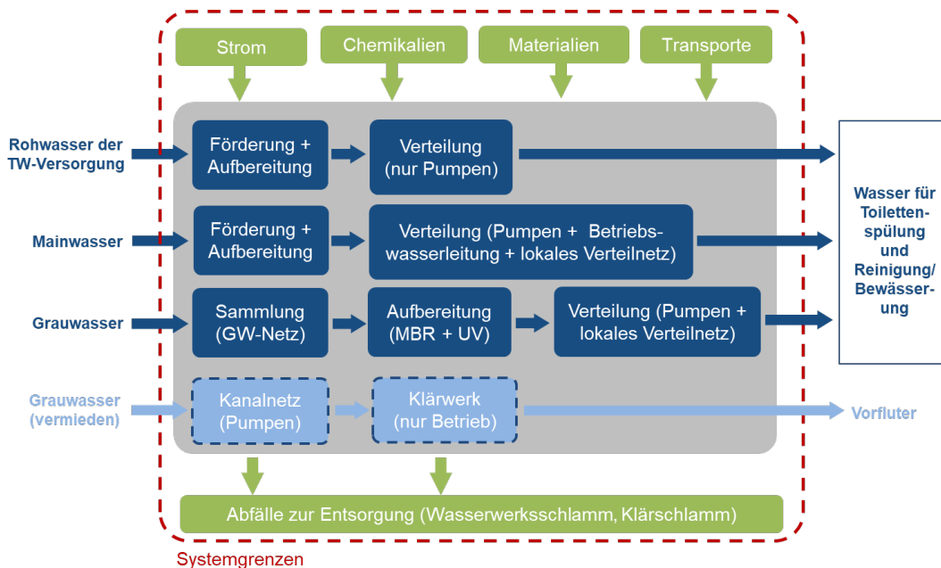
Abbildung 16: Systemgrenzen der Bilanzierung für den CO 2 -Fußabdruck
