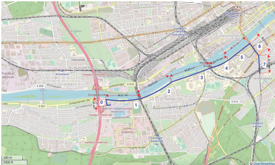
Abbildung 31: Lage der Transportleitung MWA-Heimatsiedlung Basierend auf OpenStreetMap
