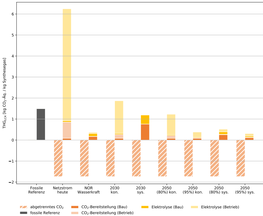
Abbildung B.19: Spezifische Treibhausgasemissionen (THG LCA ) der Bereitstellung von 1 kg CO 2 im Gemisch mit CO 2 (< 70 Vol.-%) und H 2 (< 5 Vol.-%) über die NT-Elektrolyse im Vergleich zur gewählten fossilen Referenz, die zur Abschätzung herangezogen wurde. [CO 2 -Quelle: DAC]
