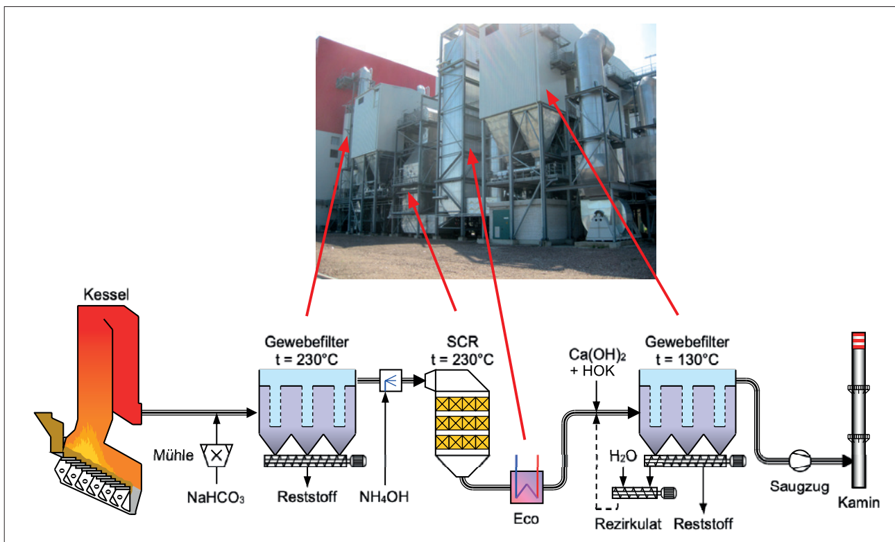
Abbildung 17: Abgasreinigung der Abfallverbrennungsanlage Delfzijl (NL) [4]
