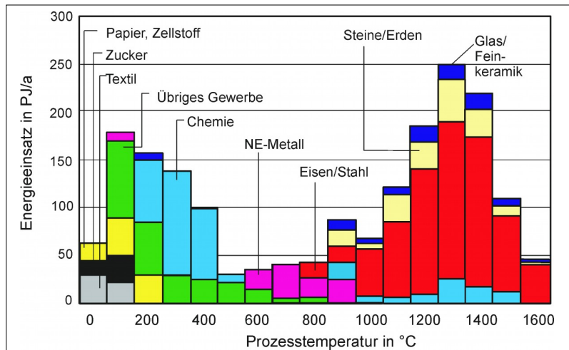
Abb. 4: Herstellungstemperaturen von Produkten [5]
