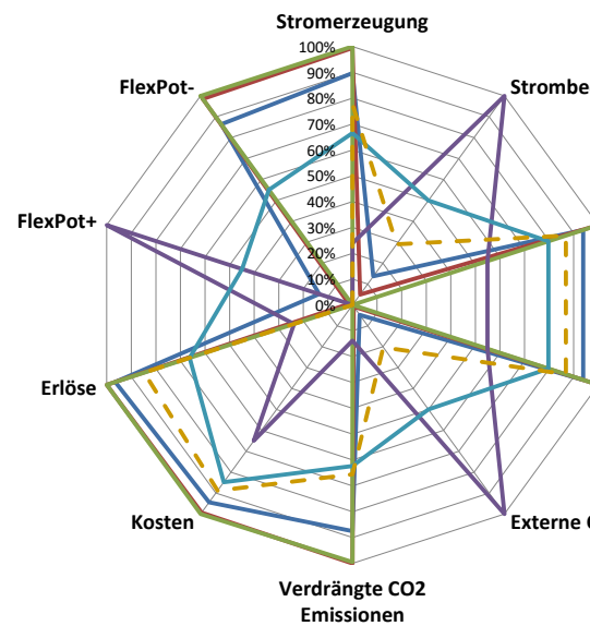
Abbildung 11.9: Verschiedene Einsatzstrategien für vollflexiblen Betrieb.
