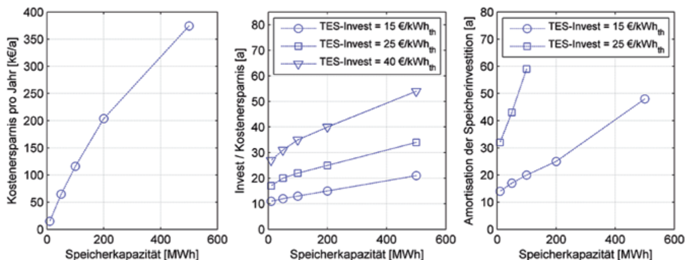
Abb. 3.5: Links: Kostenersparnis pro Jahr durch thermischen Speicher in Abhängigkeit der Speicherkapazität. Mitte: Quotient aus Investition für Speicher und Kostenersparnis pro Jahr (keine Verzinsung und Betriebskosten berücksichtigt). Rechts: Amortisation mit Verzinsung ( p = 3\% ) und Betriebskosten (1 % der Investkosten).
