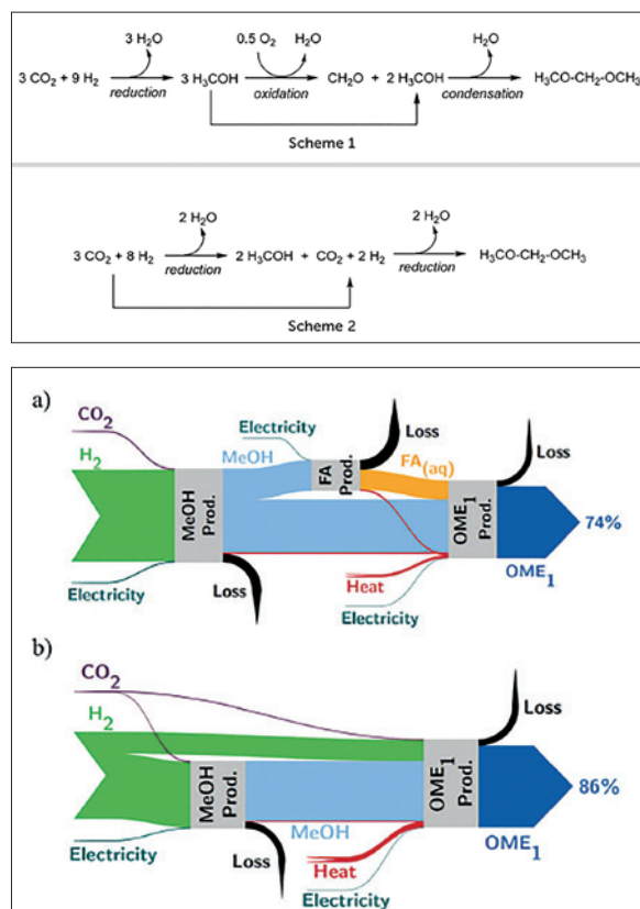
Abbildung 12: Vergleich von zwei Routen der OME 1 (oxymethylene ethers) Production (oben) und die entsprechenden Exergieflüsse (Sankey-Diagramm, unten). (© Deutz et al. 2018 ( https://dx.doi.org/10.1039/c7ee01657c ))
