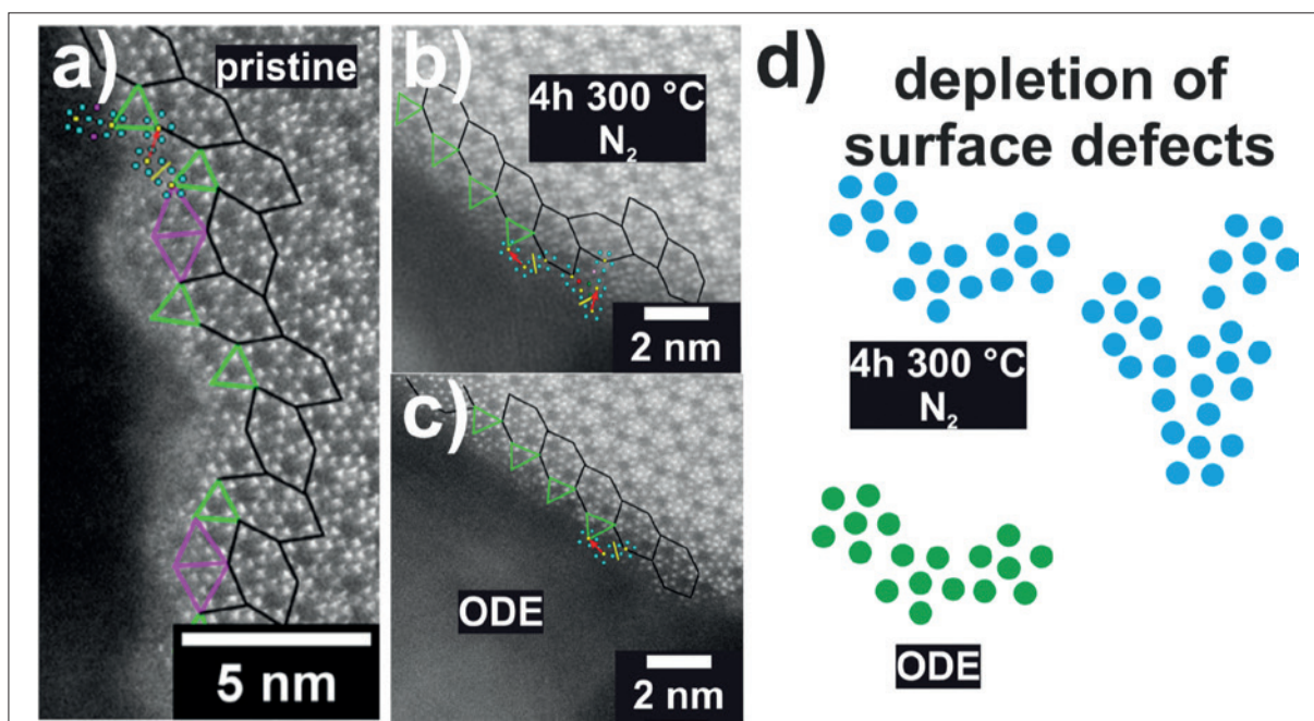
Abbildung 23: Dynamik eines kristallinen, defektreichen Mischmetalloxid-Katalysators ((Mo,V)Ox - M1 Phase) für die oxidative Dehydrierung von Ethan zu Ethylen, untersucht mittels hochaufgelöster quasi-in-situ Dunkelfeld-Rastertransmissionselektronenmikroskopie an identischen Stellen des a) hydrothermal synthetisierten Materials, b) nach thermischer Behandlung in N 2 -Atmosphäre bei 300 °C für 4 h, und c) nach oxidativer Dehydrierung von Ethan (ODE); Die verschieden farbigen geometrischen Figuren sollen die Veränderungen von Strukturmotiven der M1 Phase veranschaulichen; In d) ist die Umwandlung von Oberflächendefekten während der Reaktion schematisch dargestellt. (© Trunschke/Schunk)
