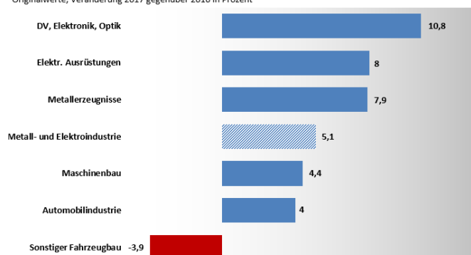
Auftragseingänge in den Branchen der M+E-Industrie Originalwerte, Veränderung 2017 gegenüber 2016 in Prozent
