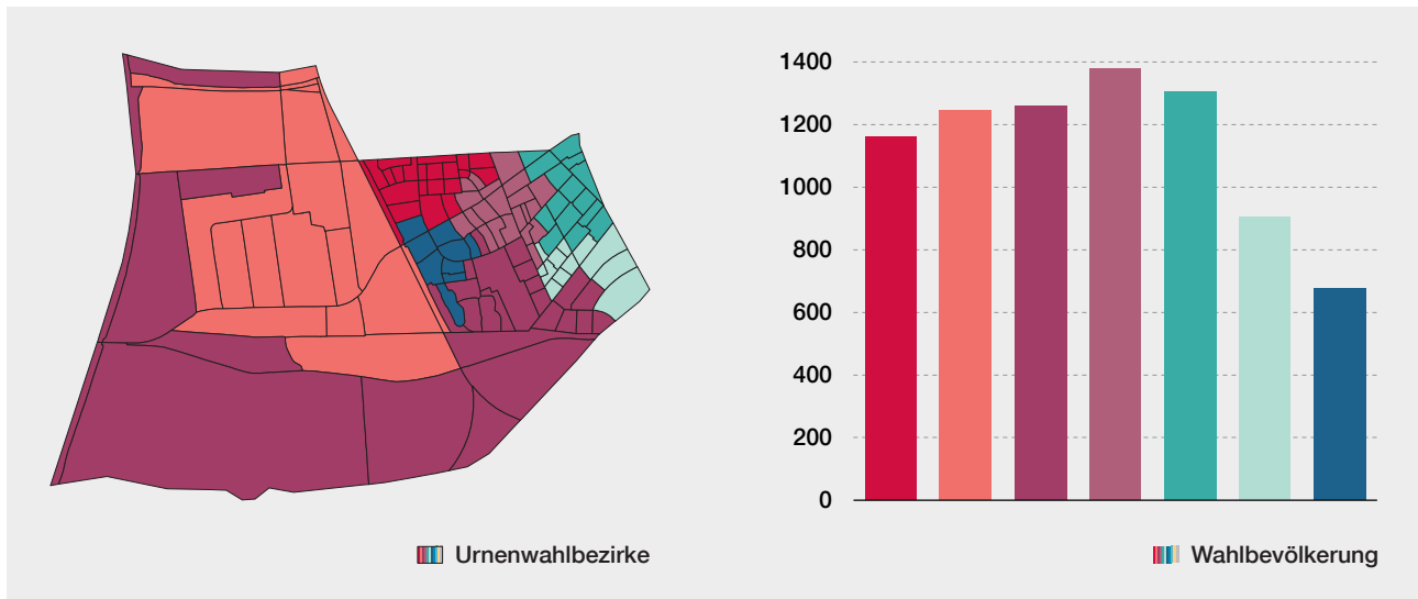
Abb. 10 Beispiel ungeeigneter Wahlbezirkseinteilung
