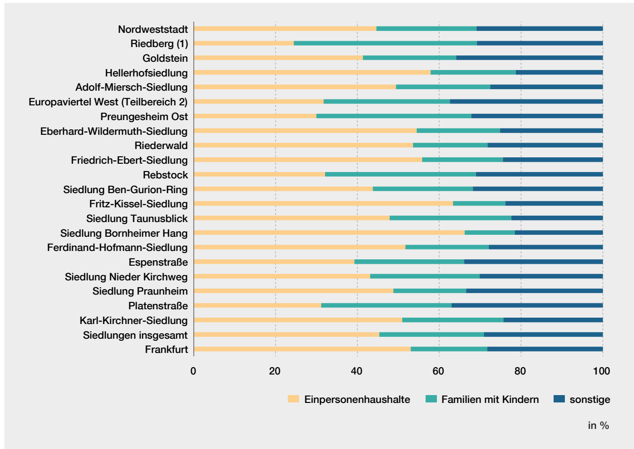
Abb.2 Haushalte in Frankfurter Siedlungen 2020
