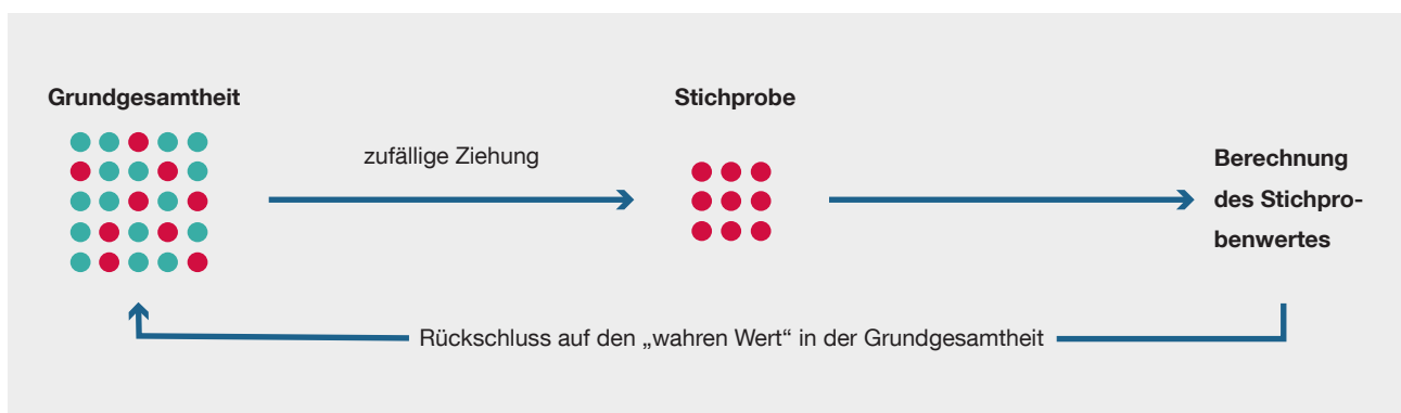
Abb. 1 Beziehung von Grundgesamtheit und Stichprobe
