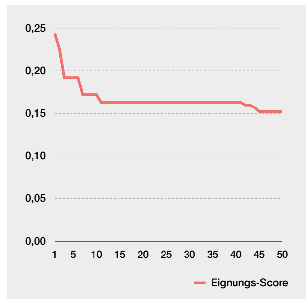
Abb. 8 Typische Entwicklung eines Eignungs-Scores
