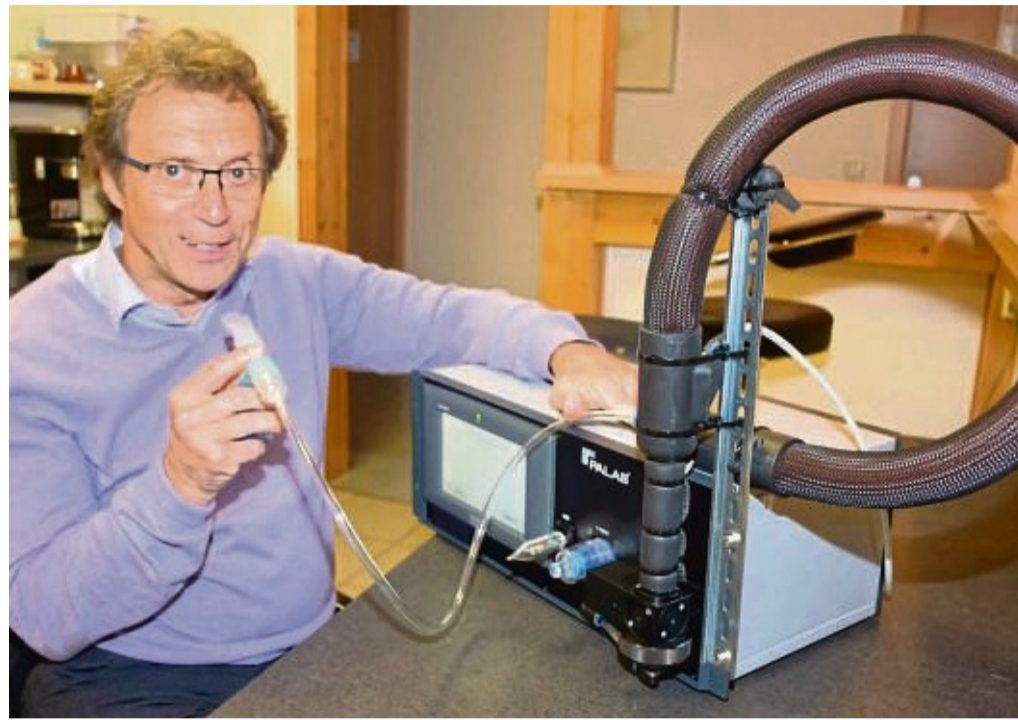
Ein Meilenstein der Aerosolforschung und Basis verschiedener Studien zur Corona-Infektion ist das 2020 von dem Gemeindeforscher Dr. Gerhard Scheuch entwickelte Resp-Aer-Meter.
