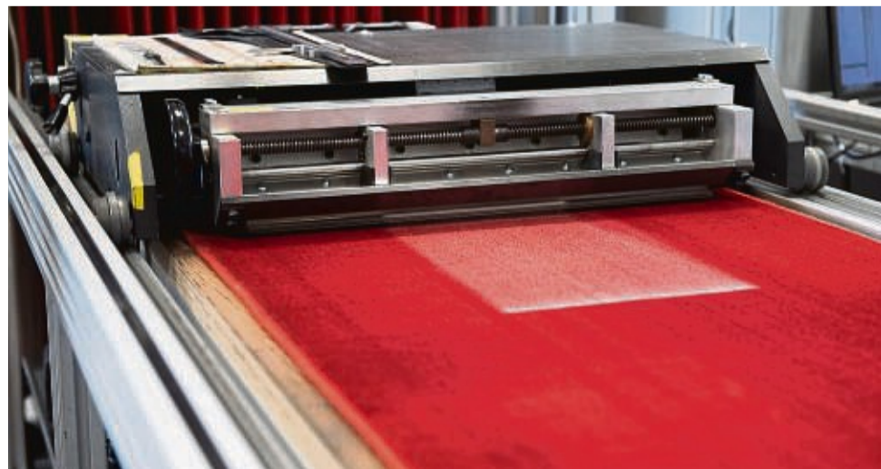
Das sind 25 Gramm Prüfstaub. Eine Maschine arbeitet sie nach festen Vorgaben in den Prüfteppich ein. So ein Teppichexemplar ist nach Angaben der Institutsmitarbeiter mehrere Tausend Euro wert - neben dem Anschaffungspreis von rund 500 Euro kommt die Summe vor allem durch die Arbeitsstunden zustande, die in die Vorbereitung des Teppichs für die Untersuchungen fließen.
