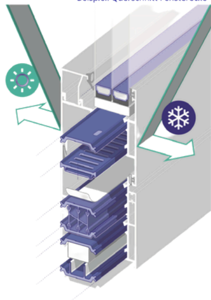
Beispiel: Querschnitt Fensterecke
