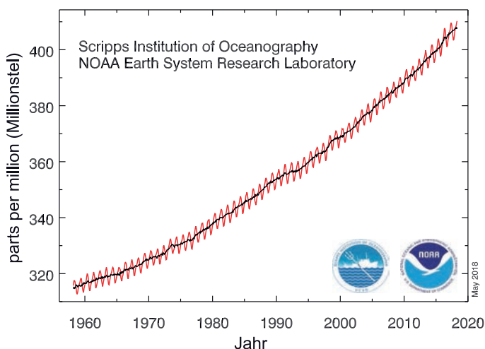
◀ Mittlere Konzentration des atmosphärischen CO 2 , gemessen am Mauna Loa Observatorium (Hawaii). Die Daten bilden die weltweit längste Reihe direkter Kohlendioxidmessungen. Dargestellt sind die Monatswerte (rote Kurve) sowie Jahresmittel (schwarze Kurve). Die Schwankungen innerhalb eines Jahres sind durch die unterschiedlichen Wachstumsperioden der Vegetation bedingt. (Quelle: NOAA)
