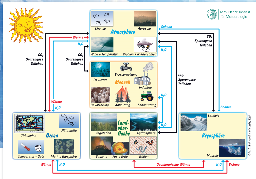
▲ In einem Klimamodell werden die wesentlichen Prozesse und Wechselwirkungen in der Natur mit Nährungsformeln beschrieben. Einige der Wechselwirkungen sind hier dargestellt. (Quelle: Max-Planck-Institut für Meteorologie)
