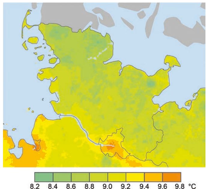
▲ Jahresmitteltemperatur in Schleswig-Holstein im Zeitraum 1981–2010 als Flächendarstellung der Rasterwerte (1 km x 1 km).
