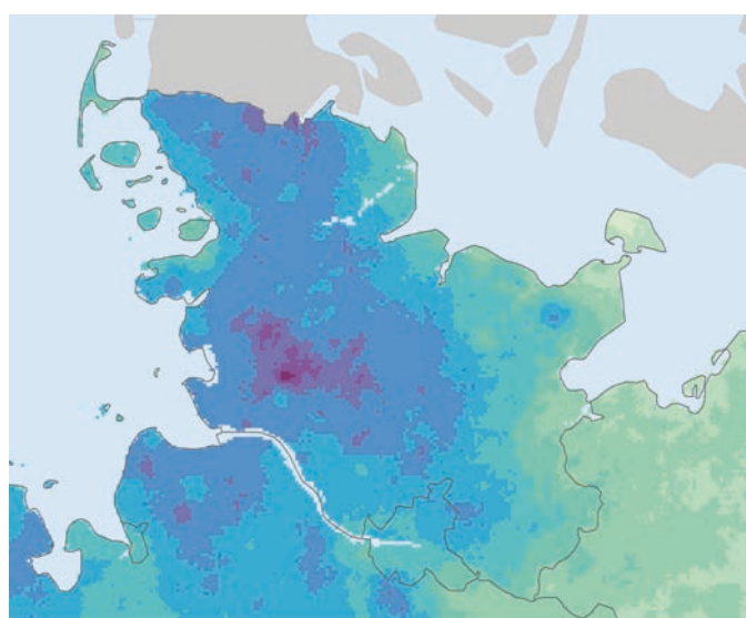
▲ Jährliche Niederschlagshöhe in Schleswig-Holstein im Zeitraum 1981-2010 als Flächendarstellung der Rasterwerte (1 km x 1 km).
