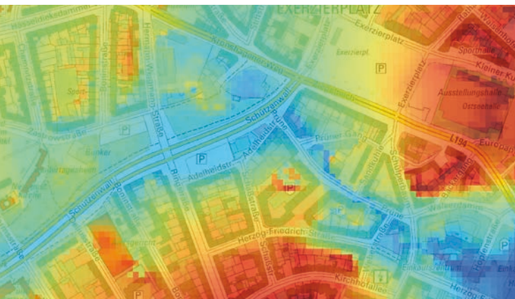
▲ Ausschnitt einer Reliefklassifikationskarte nach dem topographischen Klassifikationsindex für Flachland. Blaue Farben kennzeichnen Senken, an die bei Starkregen erhöhte Anforderungen an die Entwässerung gestellt werden. (Quelle: LLUR)
