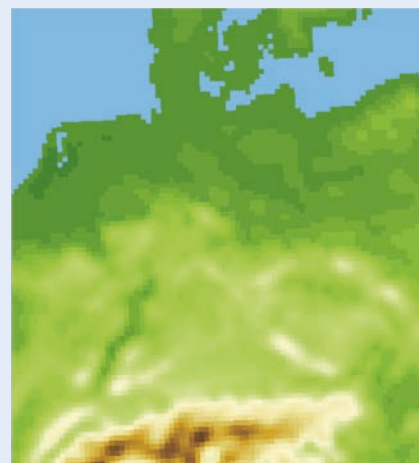
Regionales Klimamodell (fein) 0,11° (ca. 12,5 km)
