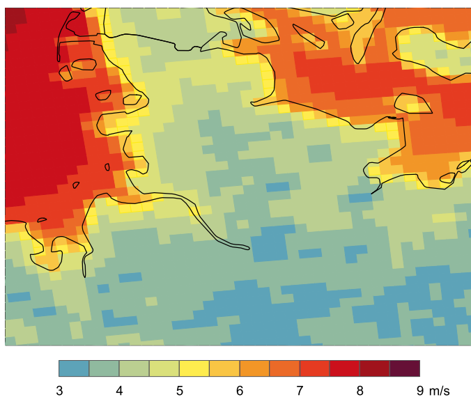
▲ Jahresmittel der Windgeschwindigkeit (10 m über Grund) in Schleswig-Holstein im Zeitraum 1995–2014 als Flächendarstellung der Rasterwerte (6 km x 6 km). Basis sind Reanalysedaten des Wettervorhersage-Modells COSMO.
