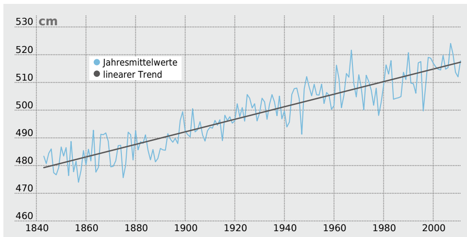
Mittlerer Meeresspiegel am ► Pegel Cuxhaven 1843–2011. (Quelle: Universität Siegen)
