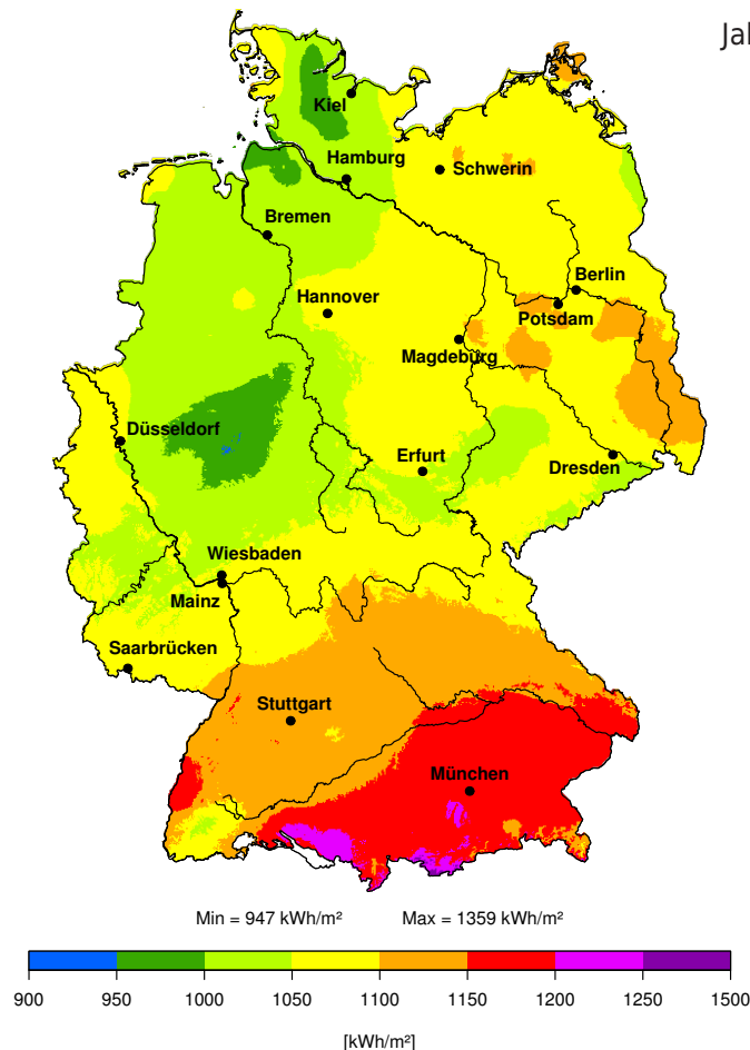
Abb. 1: Globalstrahlungskarte 2016
