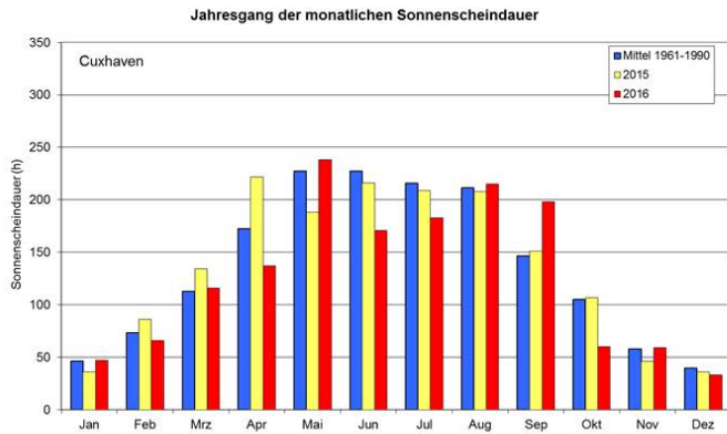
Abb. 3: Jahresgang der Sonnenscheindauer in Cuxhaven und Rostock-Warnemünde
