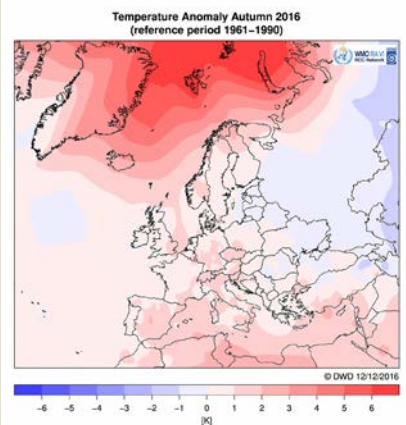
Abb. 3: Mittlere Lufttemperatur (in 2 m Höhe) in °C im Winter 2015/2016, Frühjahr 2016, Sommer 2016 und Herbst 2016 (linke Spalte) und die dazugehörigen mittlere Anomalie der Lufttemperatur (in 2 m Höhe) in K (rechte Spalte; Quelle: http://www.dwd.de/rcc-cm )
