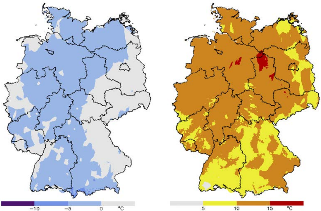
Abb. 7: Temperaturunterschiede im Mai 2016
