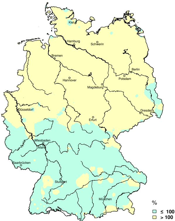
Abb. 4: Abweichung der Jahreszeit Frühling des vieljährigen Mittel 1961-1990
