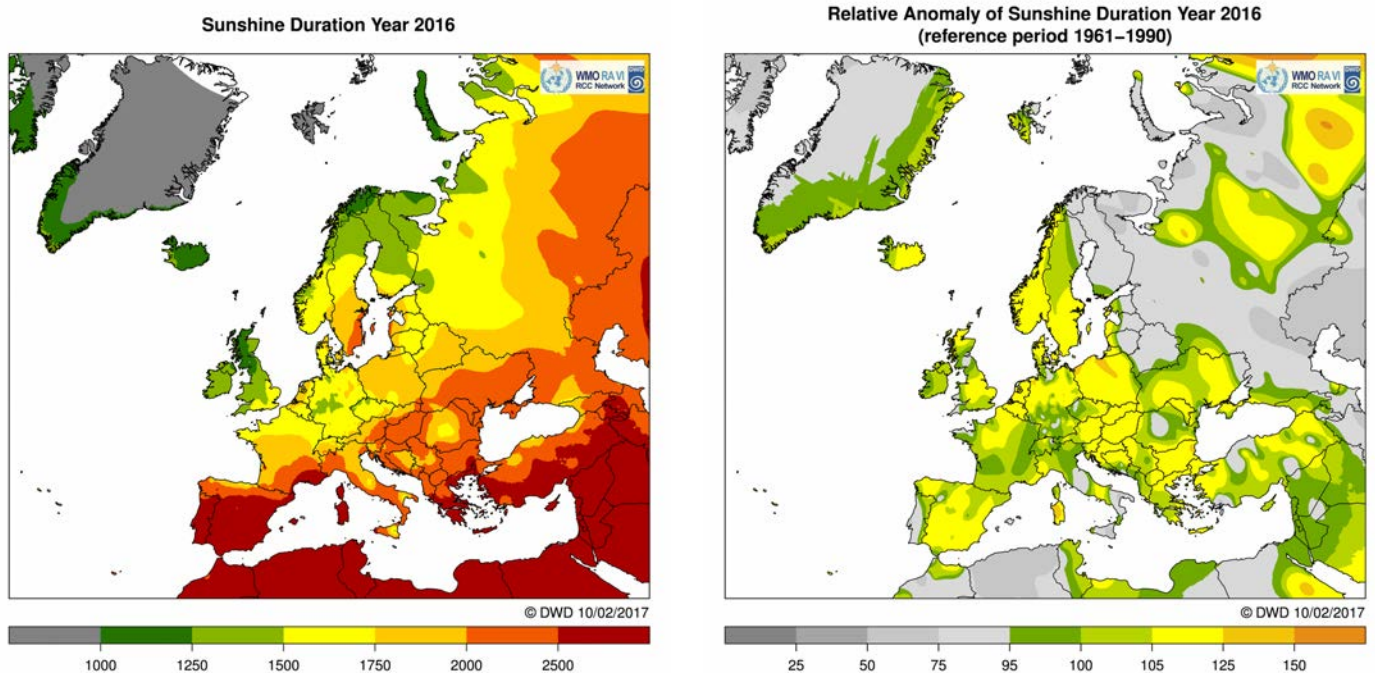
Abb. 8: Jahressumme der Sonnenscheindauer in Stunden (links) und deren relative Anomalien in % (rechts) zum vieljährigen Mittel 1961-1990 für das Jahr 2016 (Quelle: http://www.dwd.de/rcc-cm )
