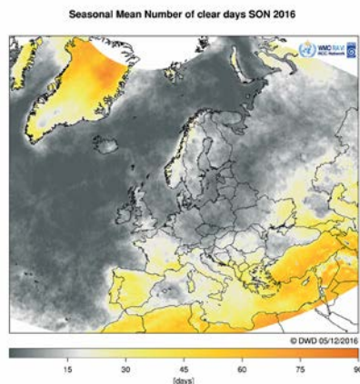
Abb. 11: Anzahl heiterer Tage (links) und deren Abweichungen (rechts) vom langjährigen Mittel 1982-2009 aus Sattelitebeobachtungen für die Jahreszeiten Winter 2015/2016, Frühling 2016, Sommer 2016 und Herbst 2016
