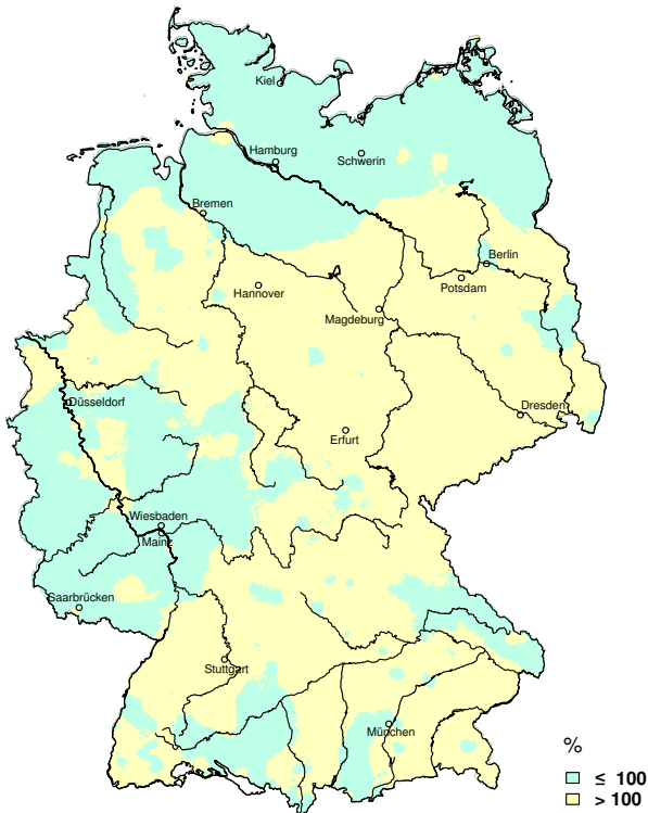
Abb. 5: Abweichung der Jahreszeit Sommer des vieljährigen Mittel 1961-1990
