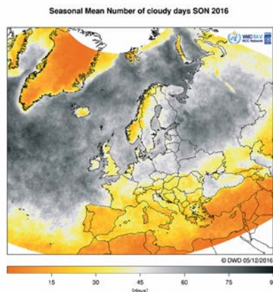
Abb. 10: Anzahl trüber Tage (links) und deren Abweichungen (rechts) vom langjährigen Mittel 1982-2009 aus Sattelitebeobachtungen für die Jahreszeiten Winter 2015/2016, Frühling 2016, Sommer 2016 und Herbst 2016
