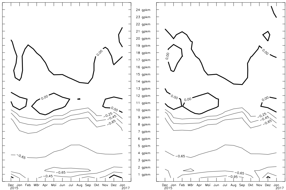
Abb. 4: Jährlicher Gang des vertikalen Gradienten der Lufttemperatur, Schleswig und Stuttgart 2016
