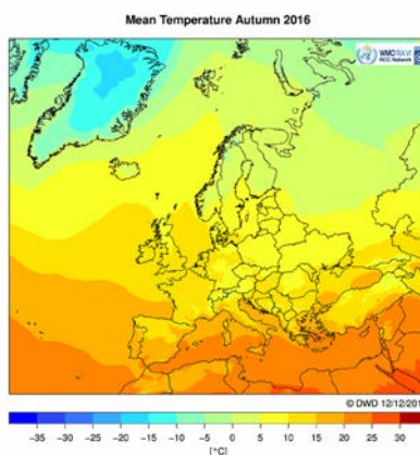
Abb. 3: Mittlere Lufttemperatur (in 2 m Höhe) in °C im Winter 2015/2016, Frühjahr 2016, Sommer 2016 und Herbst 2016 (linke Spalte) und die dazugehörigen mittlere Anomalie der Lufttemperatur (in 2 m Höhe) in K (rechte Spalte; Quelle: http://www.dwd.de/rcc-cm )
