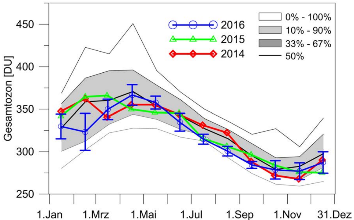
Abb. 1: Monatsmittel der Gesamtozonsäule am Hohenpeißenberg für die Jahre 2014 bis 2016. Die schattierten Bereiche geben die Perzentile der langjährigen Verteilung der Monatsmittel seit 1968 an.
