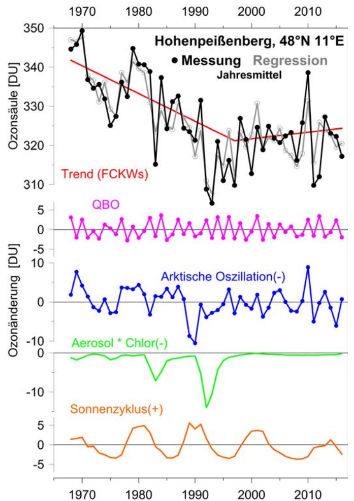
Abb.2: Oben: Jahresmittel der Gesamtozonsäule aus Messungen am Hohenpeißenberg (schwarz), sowie Rekonstruktion der Jahresmittel durch multiple lineare Regression (grau). Unten: Ozon-Schwankungen gemäß der multiplen linearen Regression: Trend durch FCKW Belastung (rot), Schwankungen durch quasi-zweijährige Oszillation der Winde am Äquator (QBO, magenta), durch meteorologische Schwankungen im Rahmen der Arktischen Oszillation (AO, blau), durch chlorgewichtete Aerosolbelastung der Stratosphäre nach Vulkanausbrüchen (grün), sowie durch Sonnenaktivität im 11-jährigen Zyklus (orange).
