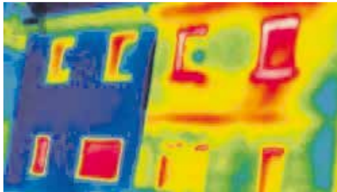
Thermographie eines Doppelhauses, links gedämmt, rechts nicht gedämmt @Copyright 2022: Energieberatung Südhessen Dr. Otterbein GmbH
