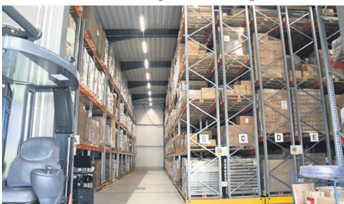
Das neue Lager ist auf einer Fläche von 25 mal 36 Quadratmetern entstanden, 8,80 Meter hoch, hat 1.900 Palettenplätze und ein effizientes Schieberegale, das eigenständig fahren kann.
