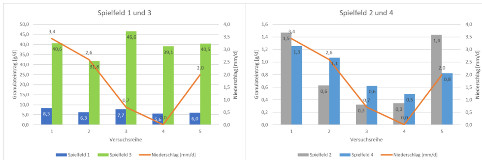
Abbildung 2: Zusammenhang zwischen Niederschlag und Eintrag von Granulat in die Niederschlagsabläufe
