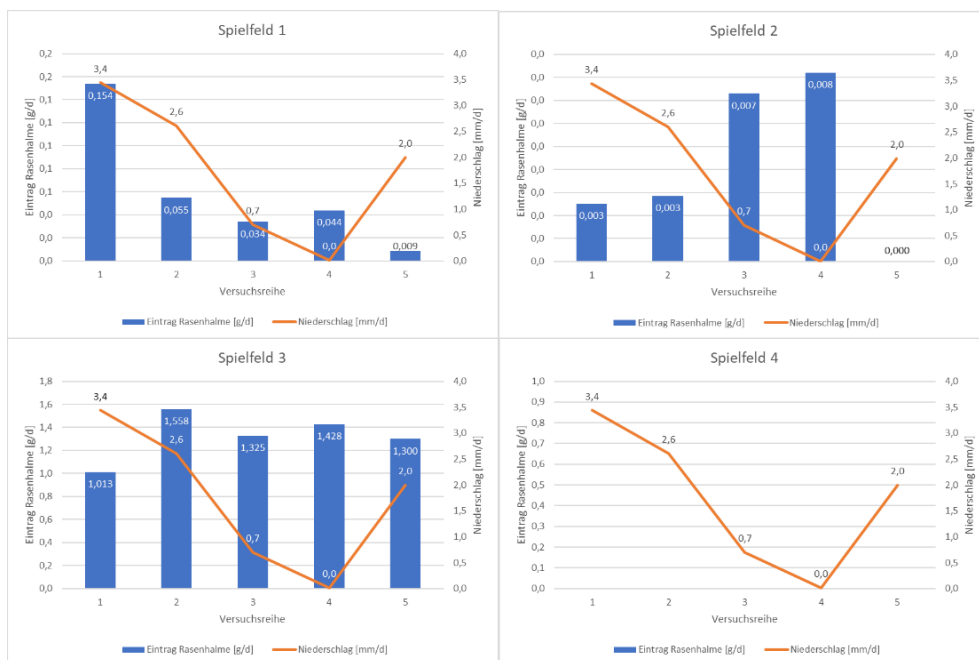
Abbildung 3: Zusammenhang zwischen Niederschlag und Eintrag von Rasenhalmen in die Niederschlagsabläufe
