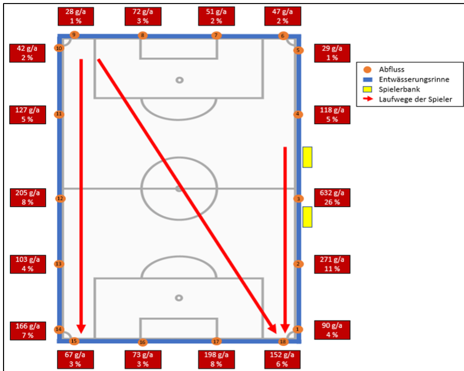
Abbildung 6: Verteilung der jährlichen Granulateinträge auf die einzelnen Abflüsse im Spielfeld 1
