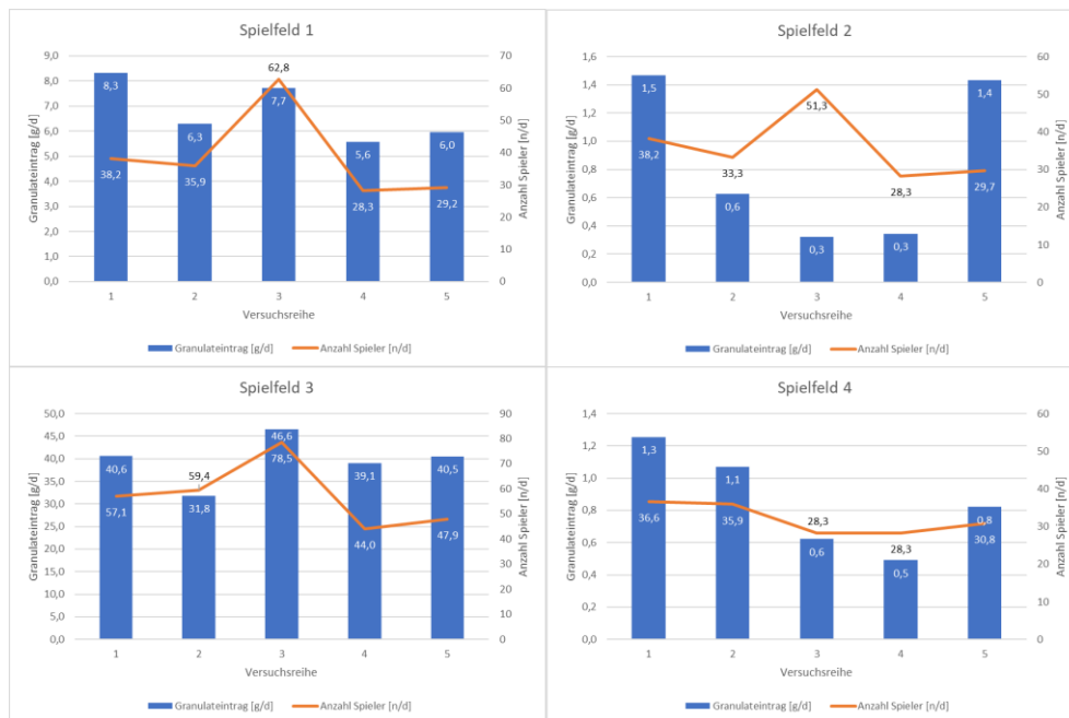
Abbildung 4: Zusammenhang zwischen Anzahl der Spieler und Eintrag von Granulat in die Niederschlagsabläufe
