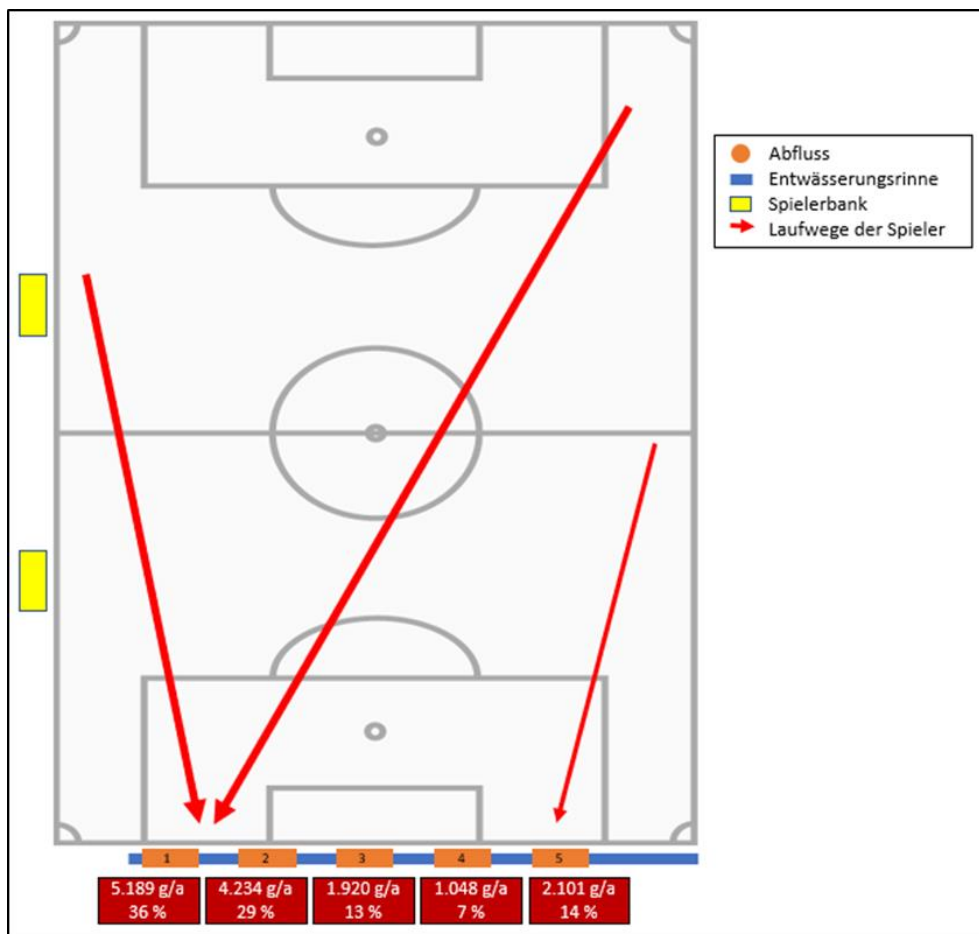
Abbildung 8: Verteilung der jährlichen Granulateinträge auf die einzelnen Abflüsse im Spielfeld 3
