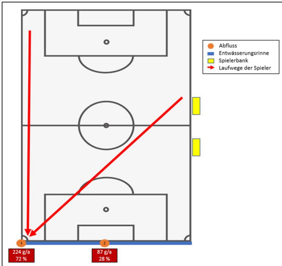
Abbildung 9: Verteilung der jährlichen Granulateinträge auf die einzelnen Abflüsse im Spielfeld 4
