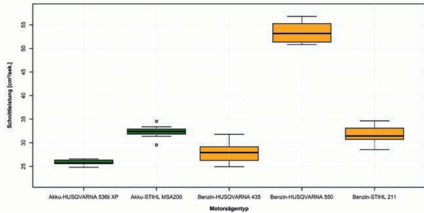
Abbildung 6: Schnittleistung in \text{cm}^2/\text{sec} der in der Studie getesteten Akku- und Benzin-Motorsägen
