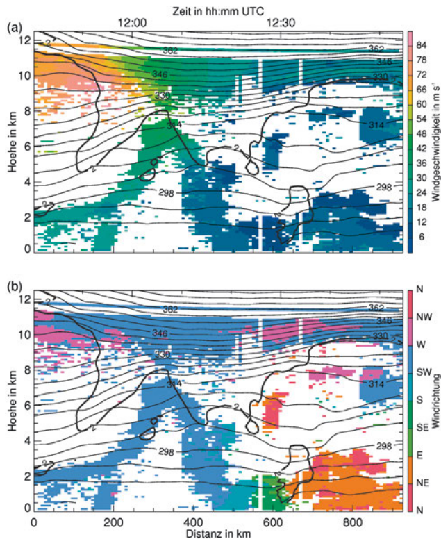
Abb. 3-6: Vom Windlidar an Bord der Falcon gemessene (a) Windgeschwindigkeit (Farbschattierung, m s^{-1} ) und (b) Windrichtung (Farbschattierung) überlagert mit der dynamischen Tropopause (2 PVU, dicke schwarze Linie) und potentiellen Temperatur (dünne schwarze Linien, K) für einen Flugabschnitt des DLR Falcon Flugs am 27. September 2016 (siehe auch Abb. 3-2b).
