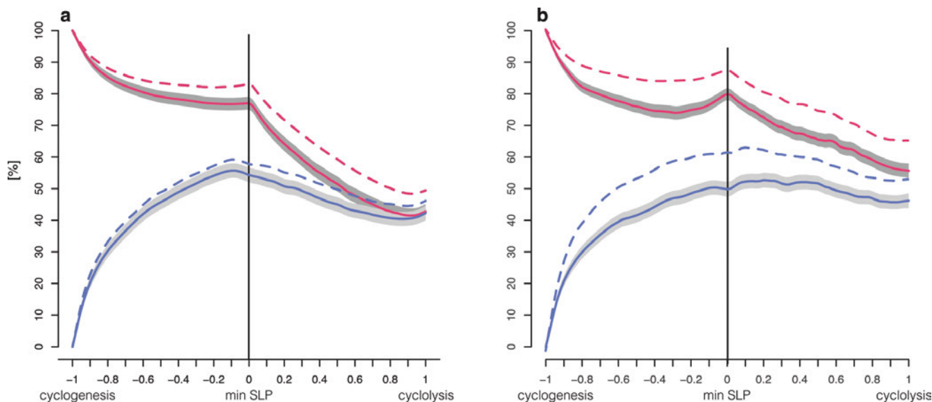
Abb. 4-8: Relativer Anteil der Zyklonen mit Fronten im Verlauf des Lebenszyklus für Zyklonen mit Front während der Zyklonogenese (rot) und ohne Front während der Zyklonogenese (blau) bei einer auf (a) äquivalent-potentieller und (b) potentieller Temperatur basierenden Frontdefinition. Die graue Schattierung entspricht dem Unsicherheitsbereich. Gestrichelte Linien entsprechen einer Frontdefinition mit reduziertem Temperaturgradienten. Der Verlauf des Lebenszyklus von Zyklonogenese bis Zyklolyse ist relativ zum tiefsten Kerndruck dargestellt (min SLP: minimum sea-level pressure ). Für Details dieser Normalisierung siehe SCHEMM et al. 2018.
