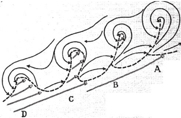
Abb. 4-1: Das vierstufige Norwegische Zyklonenmodell und die Entwicklung der Polarfront (gestrichelt). Aus BJERKNES und SOLBERG (1922).
