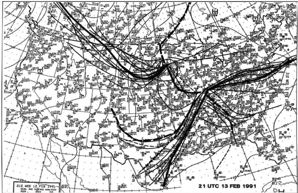
Abb. 4-2: Bodenkarte vom 13. Februar 1991 mit handgezeichneten Bodenfronten ausgewählter Experten am National Meteorological Center Workshop 25.–28. März 1991 (UCCELLINI et al. 1992).
