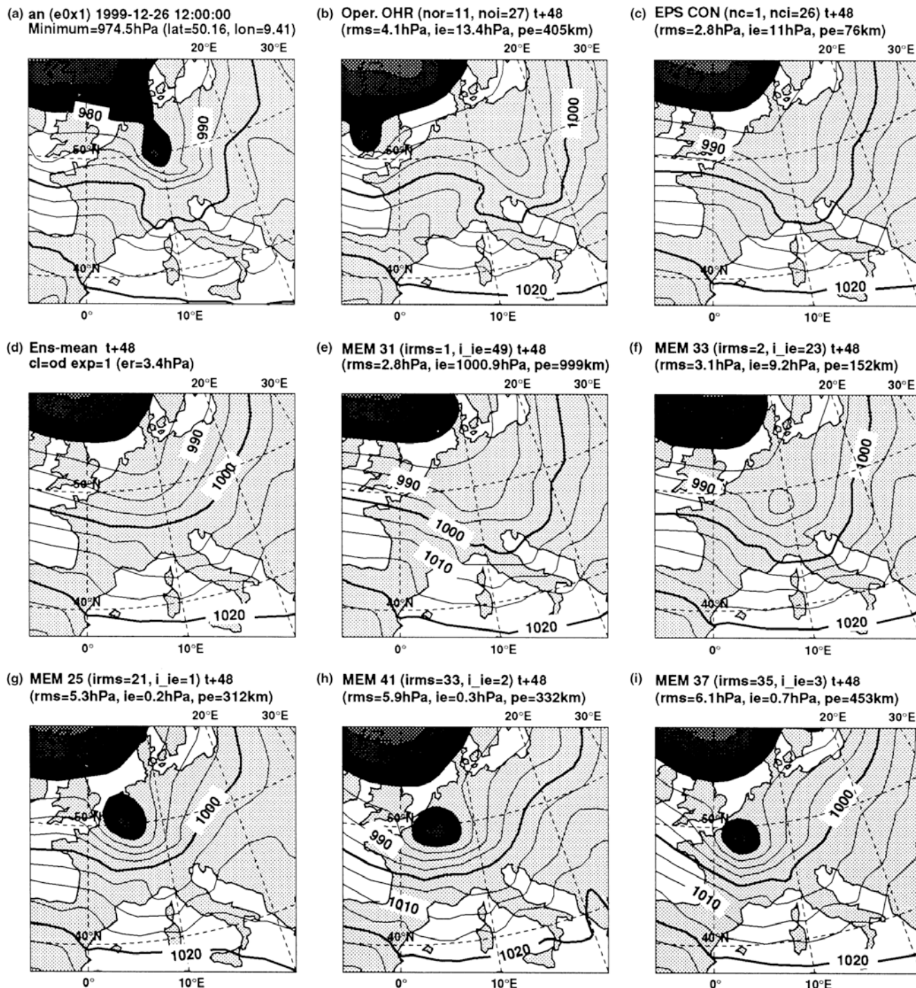
Abb. 1-2: Luftdruck auf Meereshöhe für Sturm „Lothar“ am 26. Dezember 1999 um 12 UTC nach Modellrechnungen des EZMW. Der Sturm (schwarz schattierte Fläche, Luftdruck unter 980 hPa) ist in der Analyse erkennbar (a), aber fehlt in deterministischen Vorhersagen zwei Tage im Voraus (b, c); in der Ensemble-Vorhersage wird der Sturm im Mittelwert nicht gefunden (d), jedoch in einigen der 50 Mitglieder (nicht in e, f aber in g-i). Aus BUIZZA (2002).
