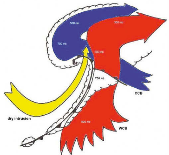
Abb. 7-2: Schematische Darstellung der drei charakteristischen Luftströmungen in einer außertropischen Zyklone: ein warmer aufsteigender Luftstrom (rot, warm conveyor belt), ein kalter aufsteigender Luftstrom (blau, cold conveyor belt) und ein trockener absteigender Luftstrom (gelb, dry intrusion). Aus CARLSON, 1980.
