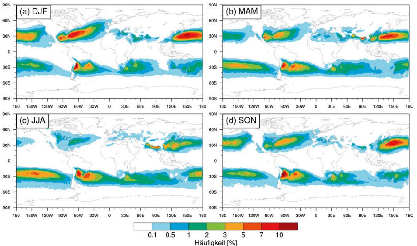
Abb. 7-4: Klimatologische Häufigkeit von WCB-Trajektorien zu Beginn ihres zweitägigen Aufstiegs für die Jahre 1979–2018 für (a) Dezember–Februar, (b) März–Mai, (c) Juni–August und (d) September–November. Die Einheit bezeichnet die Prozentzahl aller Zeitschritte mit mindestens einer WCB-Trajektorie an einem bestimmten Gitterpunkt. Reproduziert und aktualisiert von MADONNA et al. 2014.
