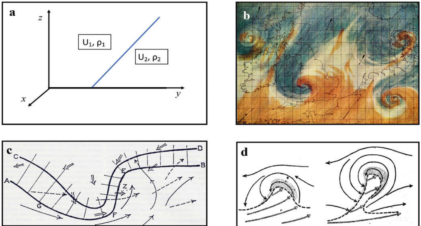
Abb. 5-3: Darstellung früherer Konzepte zur frontalen Zyklonogenese. Tafel (a) entspricht der klassischen Frontenschnittstelle von MARGULES (1906) und die nachfolgenden Tafeln zeigen schematische Darstellungen der Entwicklung von Zyklonen an einer solchen Front nach (b) FITZROY (1863), (c) EXNER (1920) und (d) BJERKNES und SOLBERG (1922).
