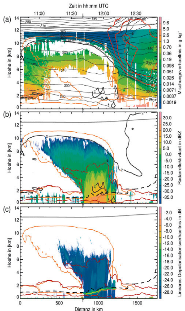
Abb. 3-4: (a) Wasserdampfmischungsverhältnis (Farbschattierung, g\ kg^{-1} ), (b) Radarreflektivität (dBz) und (c) Lineares Depolarisationsverhältnis (dB) für einen Flugabschnitt des HALO-Fluges am 26. September 2016 (siehe auch Abb. 3-2). Die graue Linie zeigt die Flughöhe. Überlagerte Konturlinien zeigen interpolierte Modellwerte des EZMW: Potentielle Temperatur (schwarze dünne Linien, K), dynamische Tropopause (2 PVU, dicke Linie), Windgeschwindigkeit (rote Linien, m\ s^{-1} ), Eiswassergehalt (orangefarbene Linie), Flüssigwassergehalt (rote Linie), 0°C Isotherme (gestrichelte schwarze Linie). Pfeile um 11:42 UTC markieren den westlichen Wendepunkt von HALO.
