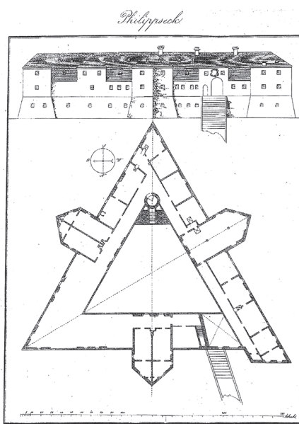
Bild 6b. Grundriss von Schloss Philippseck. Anonymer Stahlstich von 1851.
