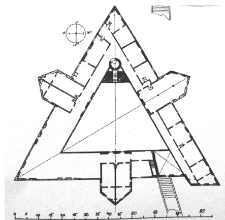
Bild 24 (vgl. Bild 6b). Dreieckiger Grundriss von Schloss Philippsseck.
