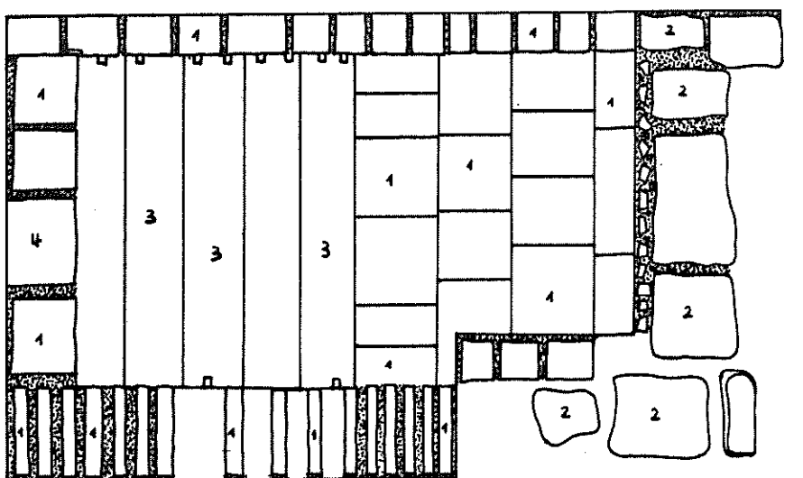
■ GRUNDRISS des Griedeler Judenbades: 1) Ziegel, 2) Basalt, 3) Eichenholz, 4) Sockel/ Wasserablauf.
