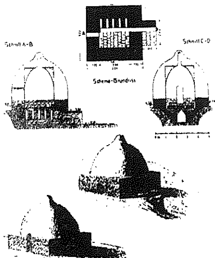
Rekonstruktion eines römischen Ziegelofens nach Ausgrabungsbefund des Landesmuseums Trier.
