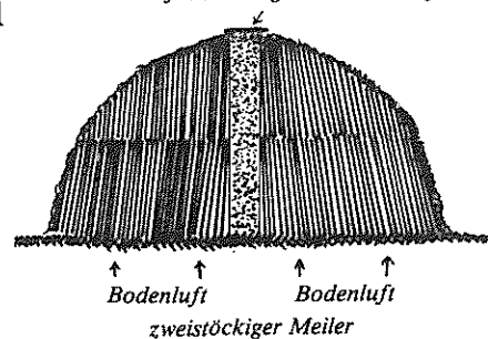
■ Funktionsschema der Meilenköhlerei, wie sie noch heute betrieben wird.
