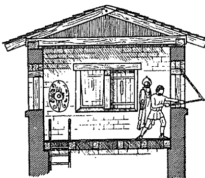
Abb. 2: ■ Schnittbild (Rekonstruktion) eines Steinturms mittlerer Größe. Für das Obergeschoß werden zwei Möglichkeiten vorgeschlagen; links mit umlaufender Außengalerie, rechts mit großem Aussichtsfenster. Seitenlänge des Turms 4,8 m. nach D. Baatz
