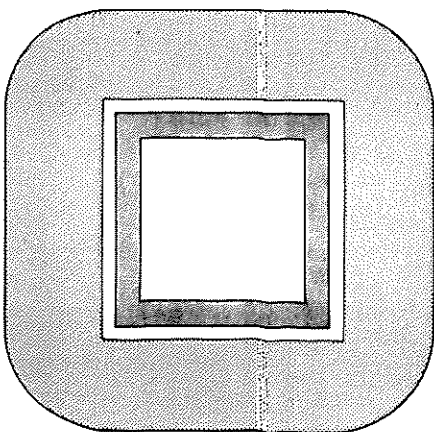
Abb. 1: ■ Grundriß und Querschnitt des Steinturms WP 4/33 auf dem Schrenzer bei Butzbach. M. 1:100
