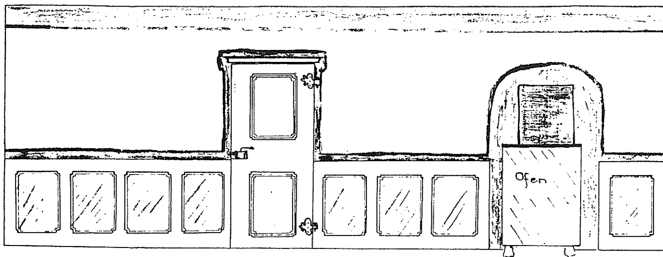
REKONSTRUKTIONSVERSUCH VON DER OST-(INNEN-)WAND DER STUBE WETZLARERSTR.13 BUTZBACH SPÄTES 18. JHT.
