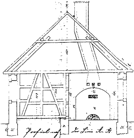
Entwurf eines neuen Backhauses für die Gemeinde Griedel von 1850
