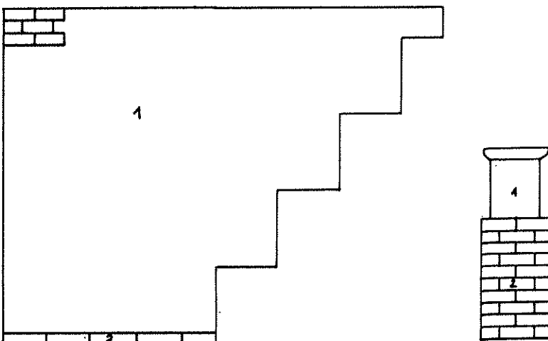
■ DAS Judenbad von Griedel in einer Auf- rißzeichnung: 1) Ziegelmauer (17 Reihen), 2) Eichenbretter.
