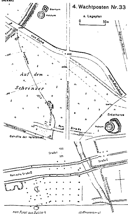
■ Plan der hallstattzeitlichen Gebäude und Gruben und der römischen Anlagen an der älteren Limeslinie („Zaungräben“) auf dem Schrenzer. Die Hallstattgebäude waren von einem Graben umgeben (nach ORL). M. 1:500.
