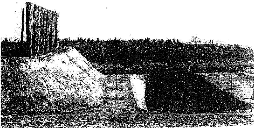
■ Rekonstruktion eines bandkeramischen Erdwerks (Graben, Wall und Palisade) nach Befunden auf der Alderhovener Platte.
