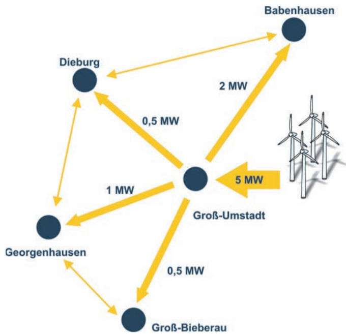
Lastverteilung des regional erzeugten regenerativen Stroms im Projekt Grid4Regio. (Grafik: ENTEGA)
