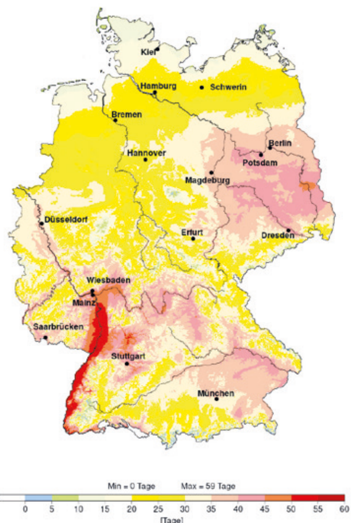
Im Oberrheintal werden die meisten Tage mit Temperaturen über 25°C gemessen. (Karte: DWD)
