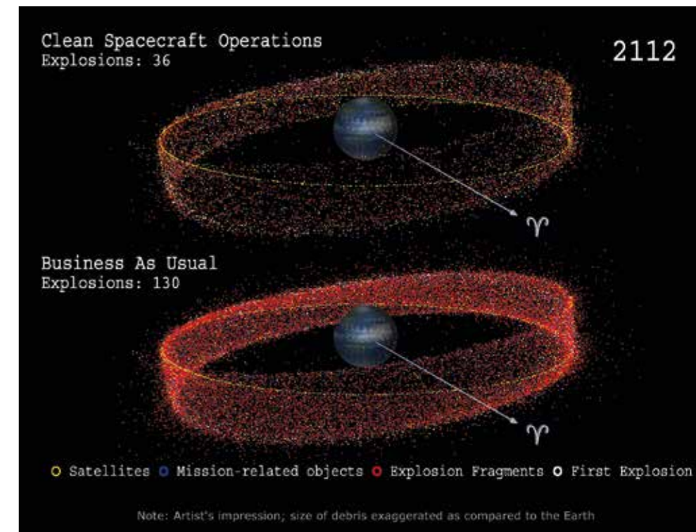
Simulation der GEO-Umgebung mit Minderungsmaßnahmen (oben) und ohne (unten). Dieses Bild zeigt eine Simulation der zukünftigen GEO-Umgebung für den Fall, dass keine Maßnahmen ergriffen werden; dies ist das „Business-as-usual“-Szenario. Im oberen Bereich ist mit Minderungsmaßnahmen eine viel sauberere Weltraumumgebung zu beobachten, wenn die Anzahl der Explosionen drastisch reduziert wird und keine missionsbezogenen Objekte ausgeworfen werden. Um jedoch die immer größer werdende Menge an Weltraumschrott zu stoppen, sind ehrgeizigere Schutzmaßnahmen erforderlich. Langfristig müssen Raumfahrzeuge und Raketenstufen nach Abschluss ihrer Mission zur Erde zurückgebracht werden. Es ist von entscheidender Bedeutung, dass wir unverzüglich mit der Umsetzung von Abhilfemaßnahmen beginnen.
