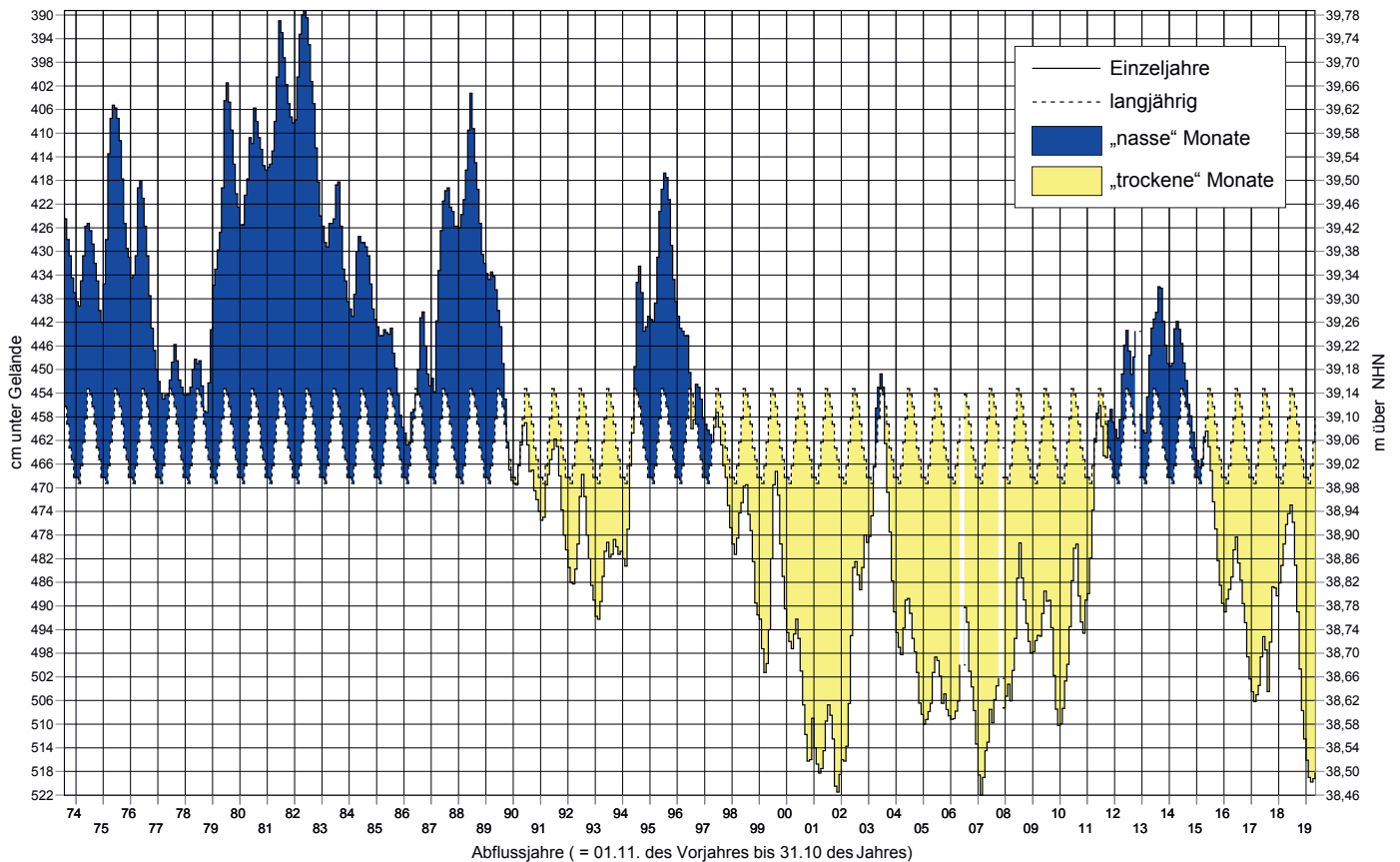
▲ Grundwasserstände in Seddin: Monatsmittel der Einzeljahre und langjährige monatliche Vergleichswerte. (Quelle: Landesamt für Umwelt Brandenburg)
