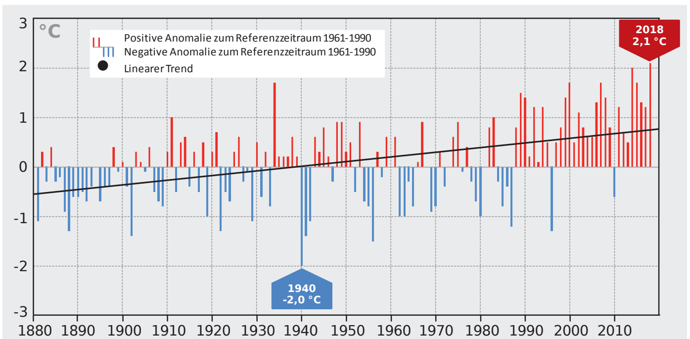
▲ Es ist wärmer geworden in Brandenburg: Abweichungen des Jahresmittels der Temperatur (Gebietsmittelwerte) 1881-2018 von der für den Referenzzeitraum 1961-1990 berechneten Jahresmitteltemperatur.
