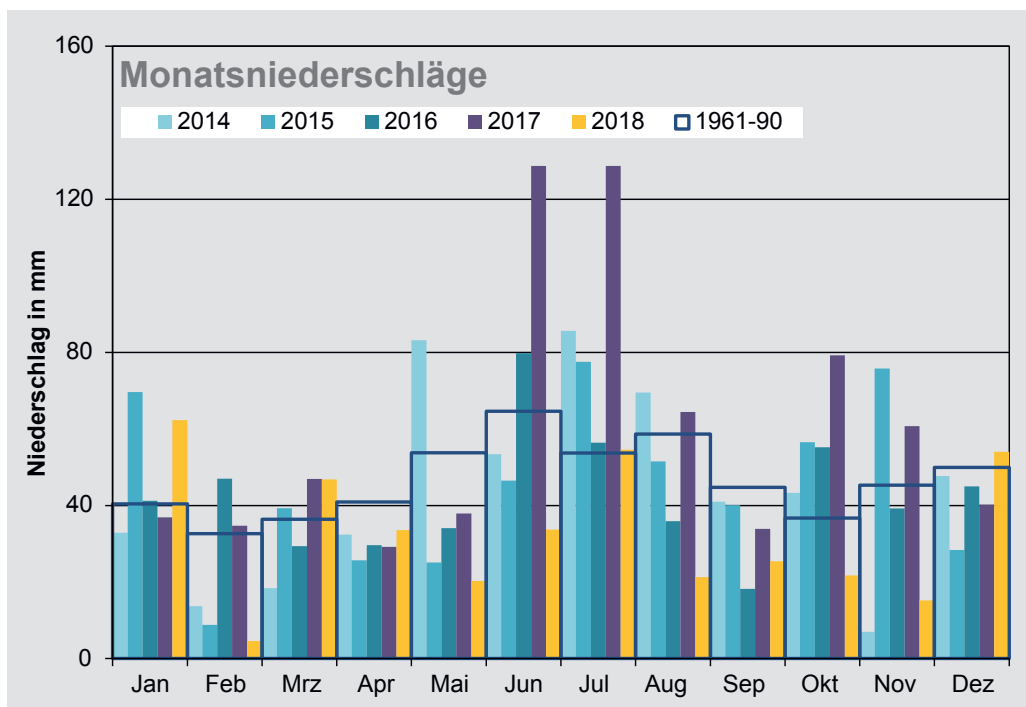
◀ Monatlicher Gebietsniederschlag in Brandenburg 2014–2018 im Vergleich zur Referenzperiode 1961–1990. (Quelle: Landesamt für Umwelt Brandenburg)
