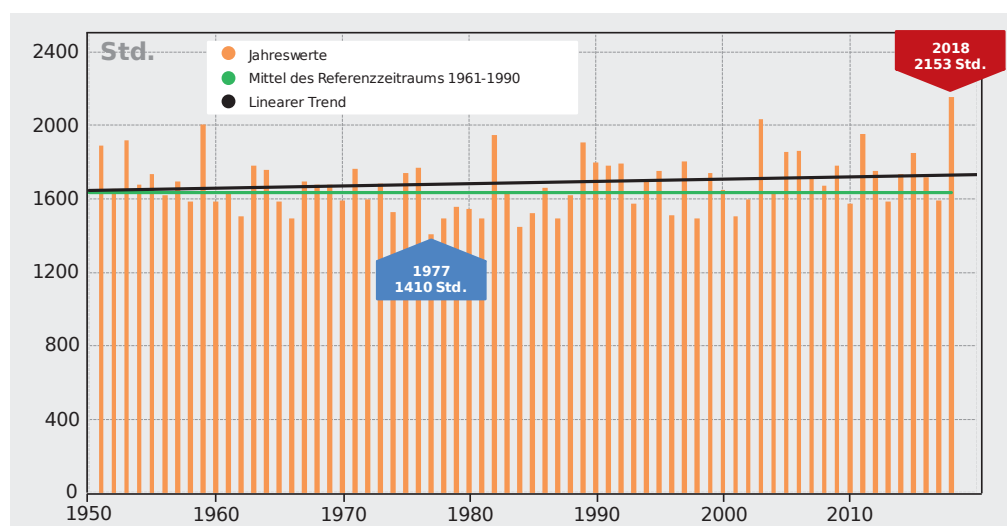
Jahressummen der Sonnenscheindauer (Gebietsmittelwerte) in Brandenburg von 1951 bis 2018.
