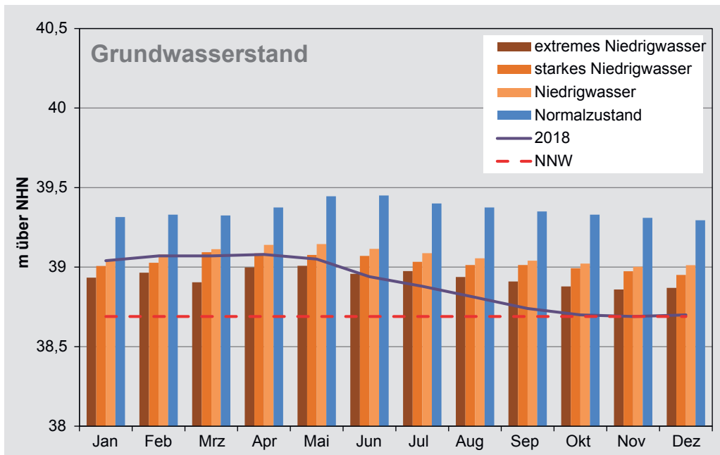
◀ Monatlicher Grundwasserstand 2018 in Beelitz - Potsdam Mittelmark. (Quelle: Landesamt für Umwelt Brandenburg)
