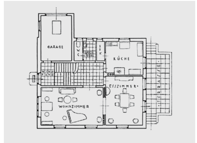
Historischer Grundriss des Erdgeschosses
